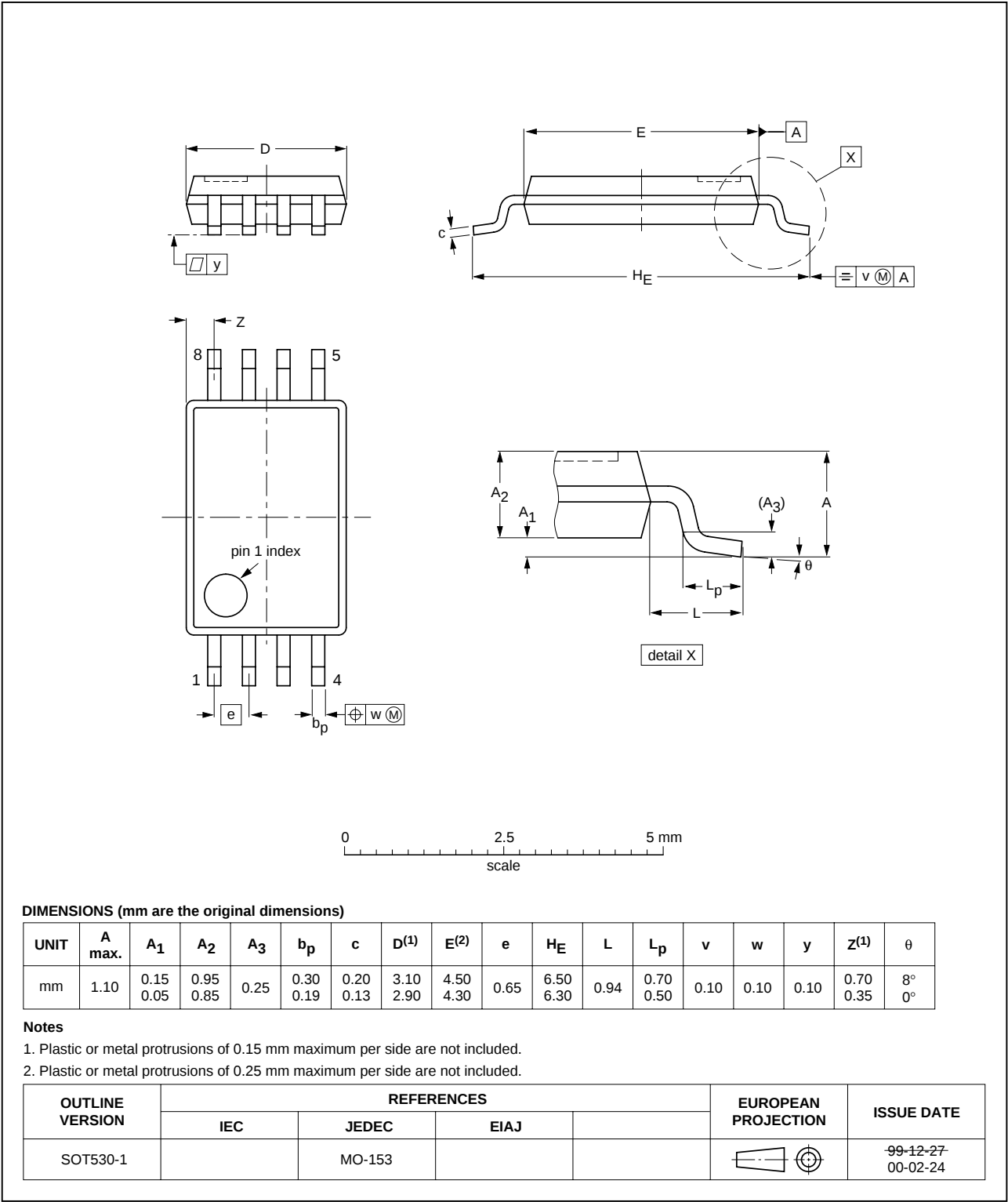
Fig 14. SOT530-1 (TSSOP8).
