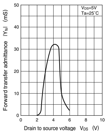
|Y_{fs}| - V_{DS}
