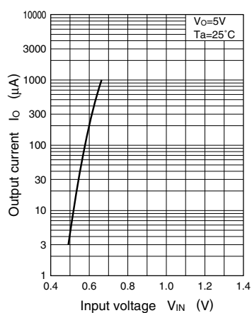
I_O - V_{IN}
