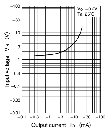
V_{IN} - I_O
