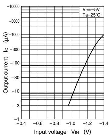
I_O - V_{IN}
