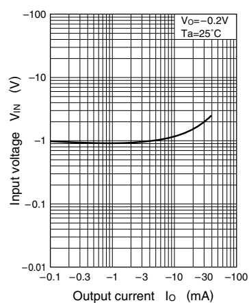
V_{IN} - I_O
