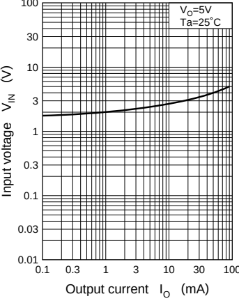
V_{IN} - I_O
