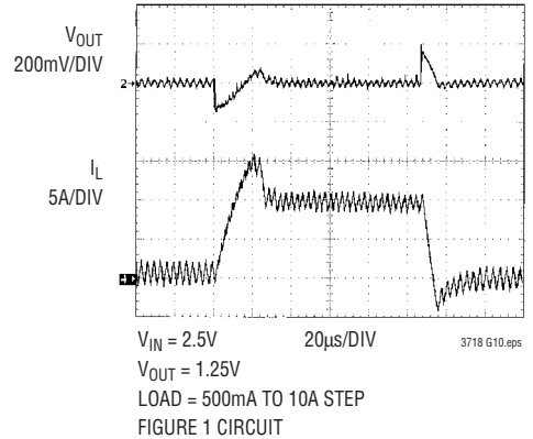
Load-Step Transient
