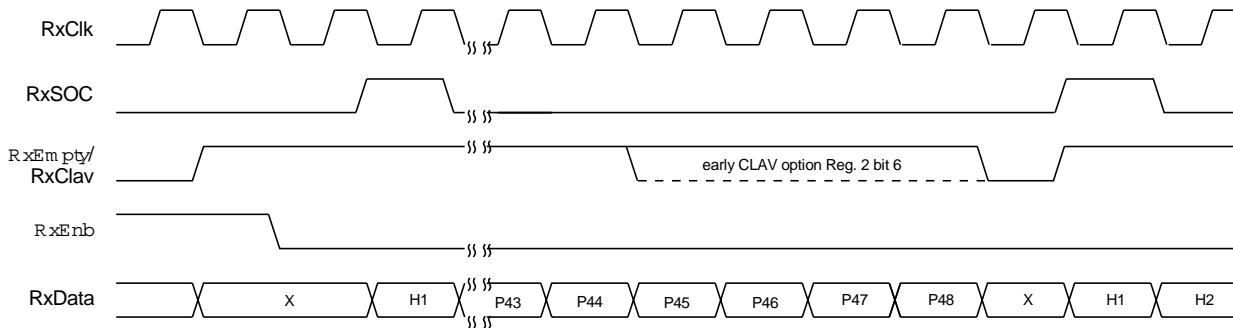
Figure 7 RxEmpty/RxClav Waveform
