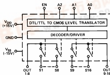
AD7507
