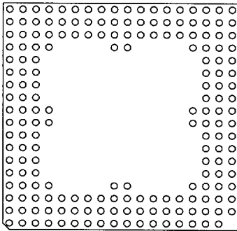
191 Pins 23
