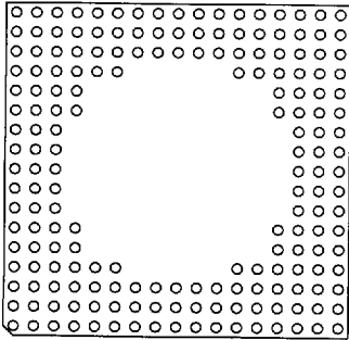
188 Pins 33
