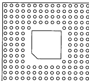
179 Pins 10
