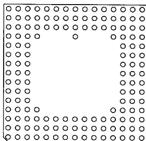
149 Pins 37
