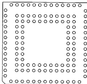
124 Pins 34
