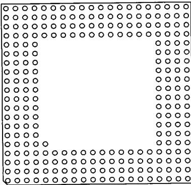
257 Pins 4
