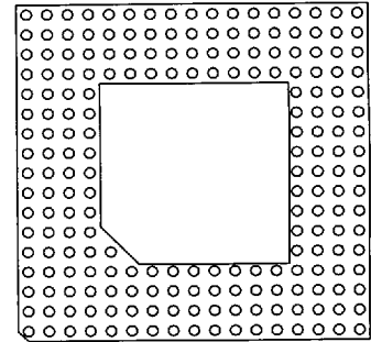
209 Pins 14
