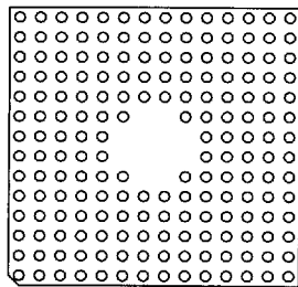
184 Pins 35
