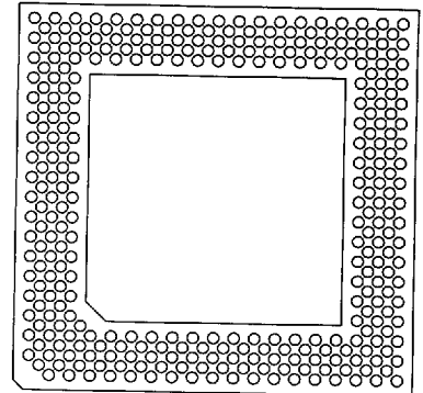
320 Pins A7 Without Window FP A5 Intel Pentium™ P54CM
