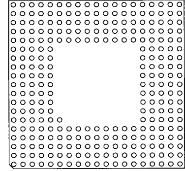
281 Pins 6
