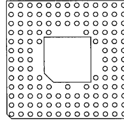
133 Pins 51
