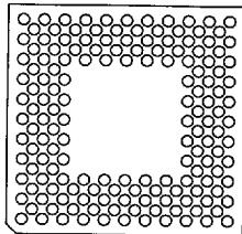
160 Pins A1
