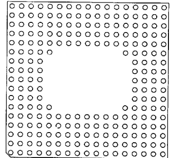
230 Pins 36
