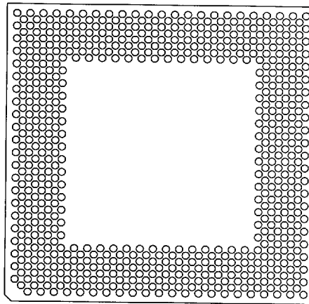
591 Pins A1
