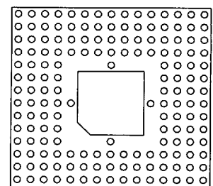
180 Pins 6
