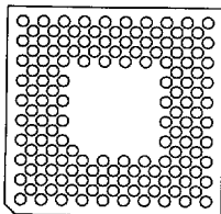
141 Pins A1
