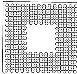
304 Pins A2
