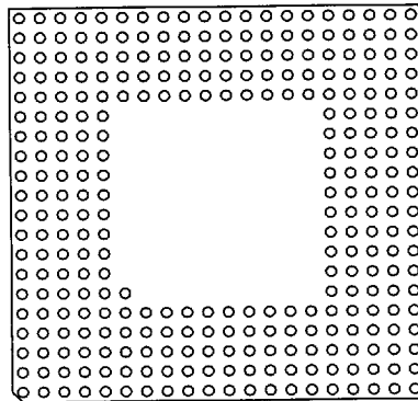
301 Pins 5
