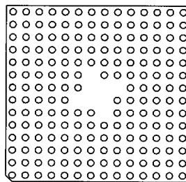
188 Pins 31
