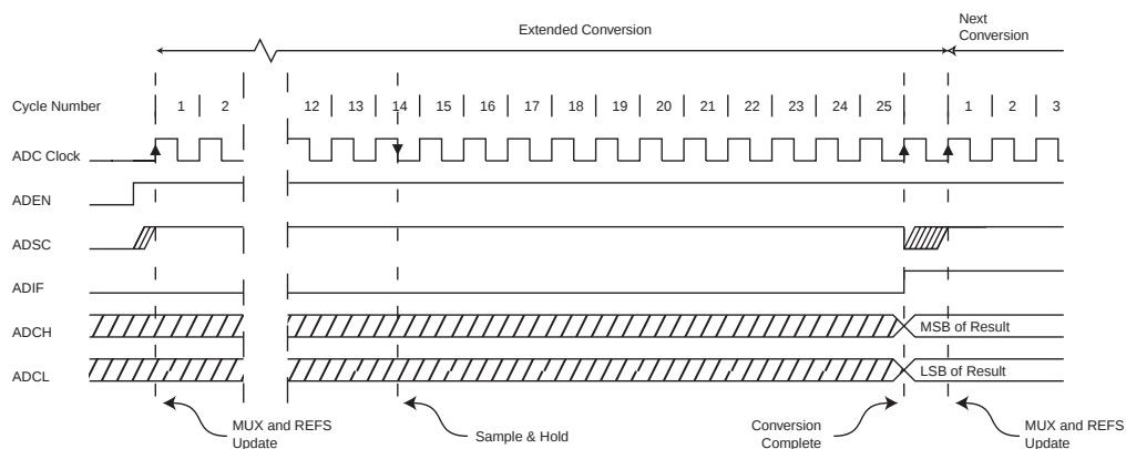
Figure 48. ADC 时序图，第一次转换 (单次转换模式)
