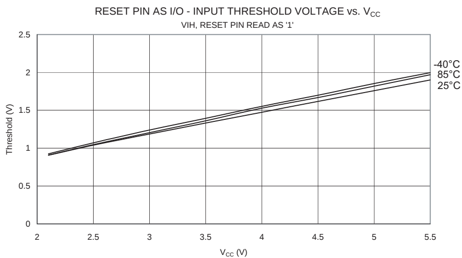
Figure 113. Reset 作为普通 I/O 输入门限电压和 V_{CC} 的关系 ( V_{IL} , Reset 引脚读值为 “0”)
