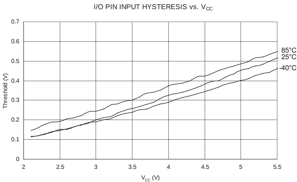
Figure 111. I/O 引脚输入迟滞和 V_{CC} 的关系
