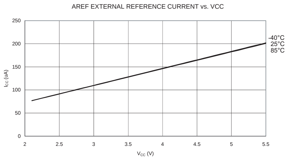
Figure 139. 模拟比较器电流和 V_{CC} 的关系
