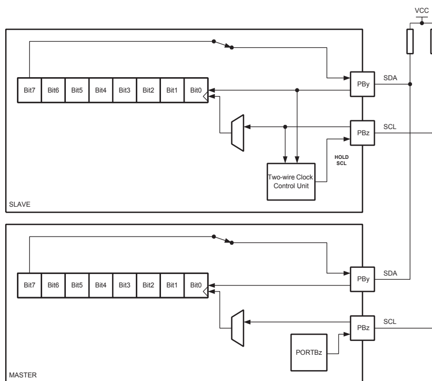
Figure 42. 两线模式框图
