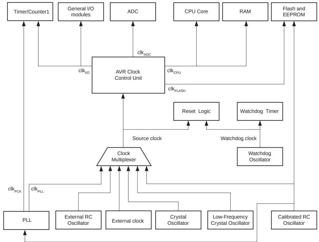
Figure 26. 时钟分布
