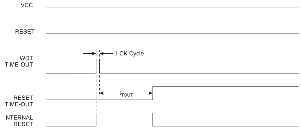
Figure 25. 看门狗溢出
