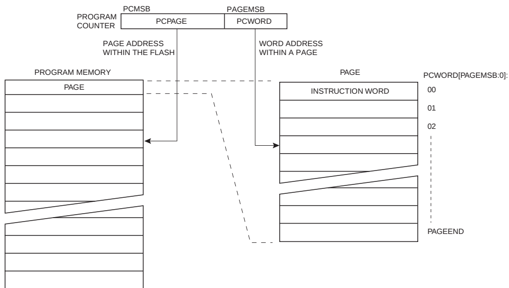
Figure 59. 对以页为组织单位的 Flash 进行寻址 (1)
