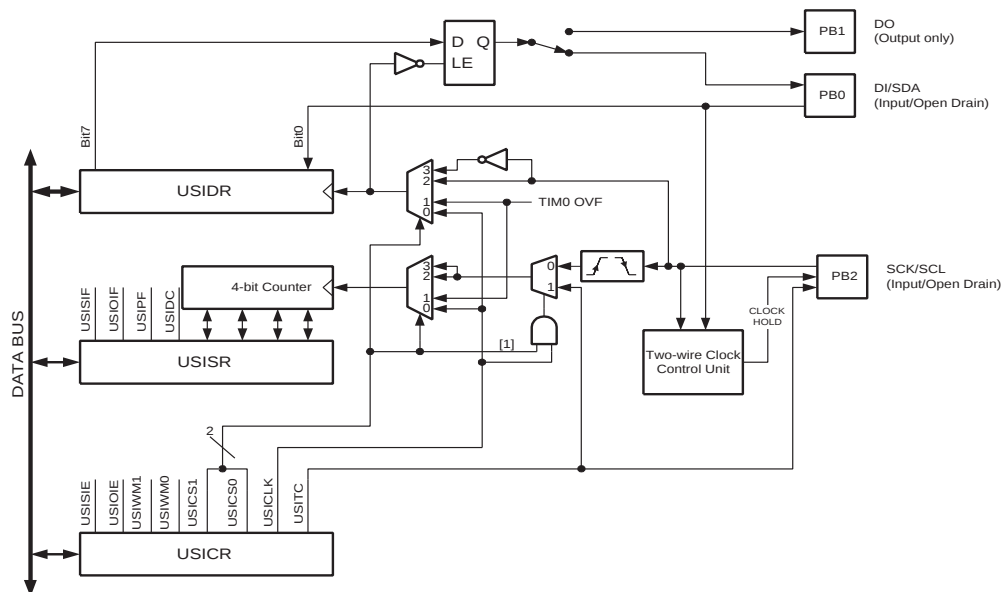
Figure 39. 通用串行接口框图
