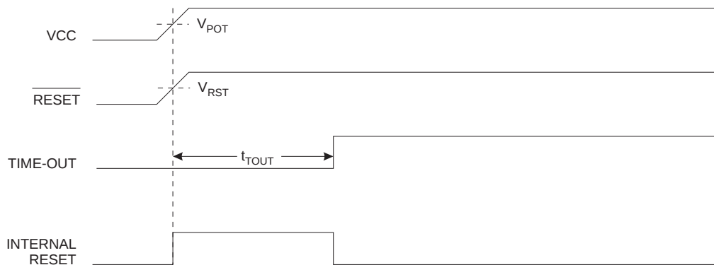
Figure 21. 通过 VCC, MCU 启动 RESET
