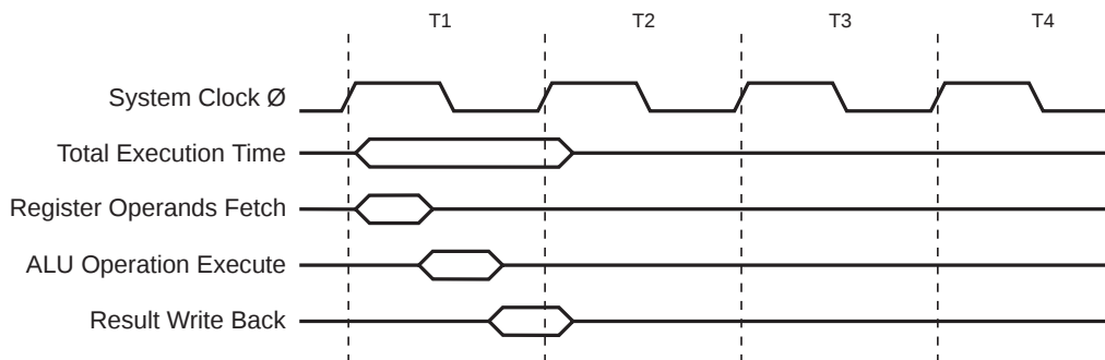
Figure 18. 单时钟周期 ALU 操作
