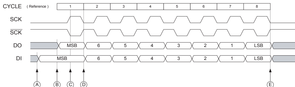
Figure 41. 三线模式时序图
