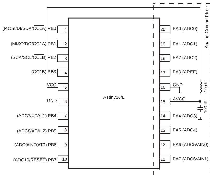
Figure 52. ADC 电源连接图
