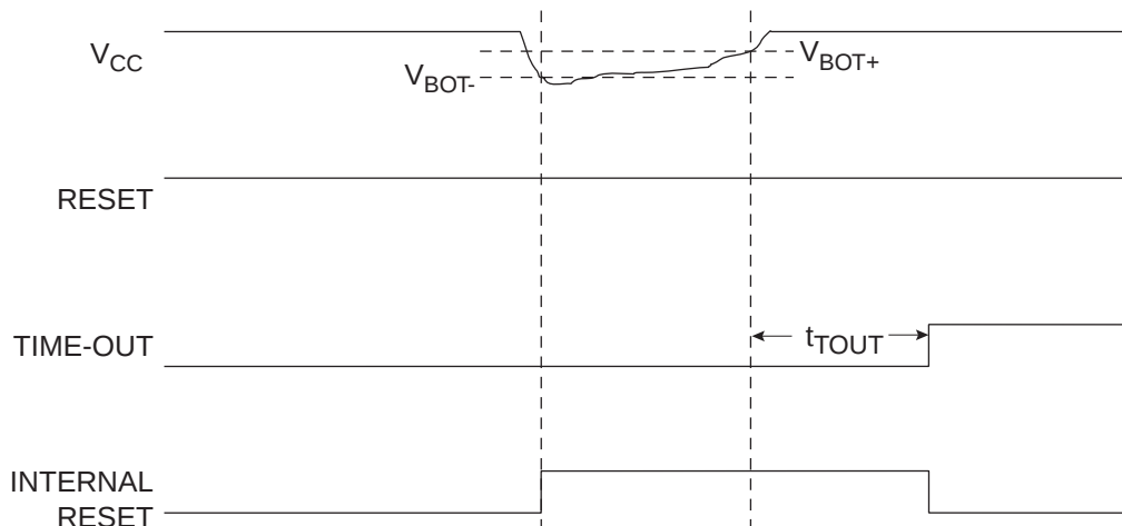
Figure 24. 运行中 BOD 复位
