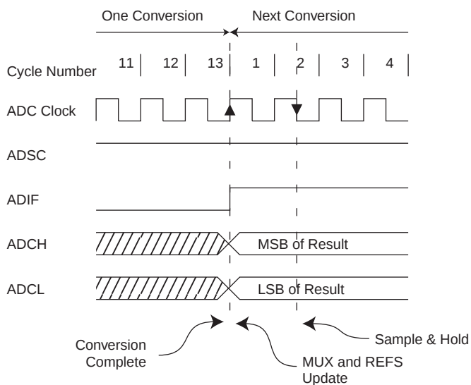
Figure 50. ADC 时序图，连续转换
