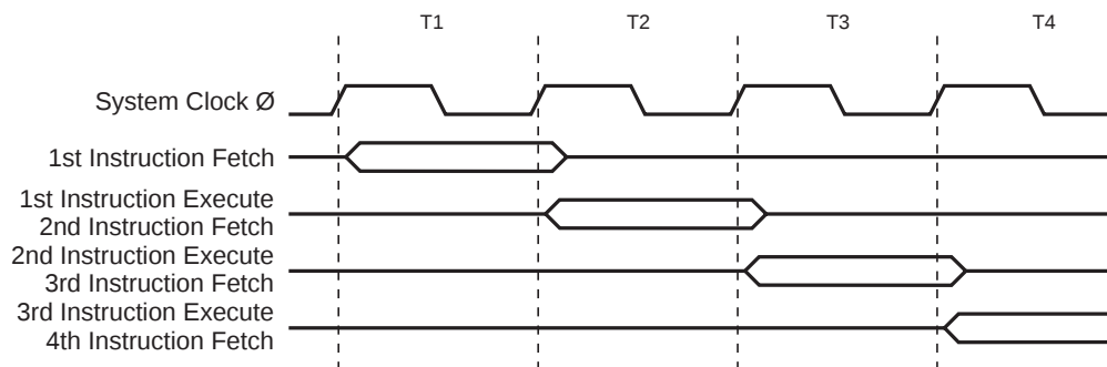
Figure 17. 并行取指和指令执行
