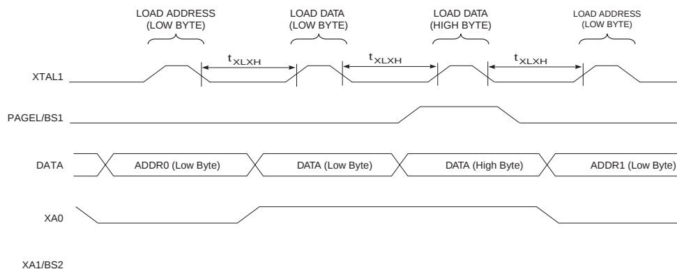
Figure 65. 并行编程时序，有时序要求的加载序列 (1)
