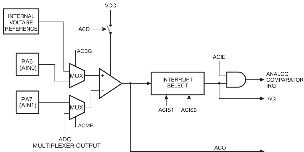
Figure 45. 模拟比较器框图
