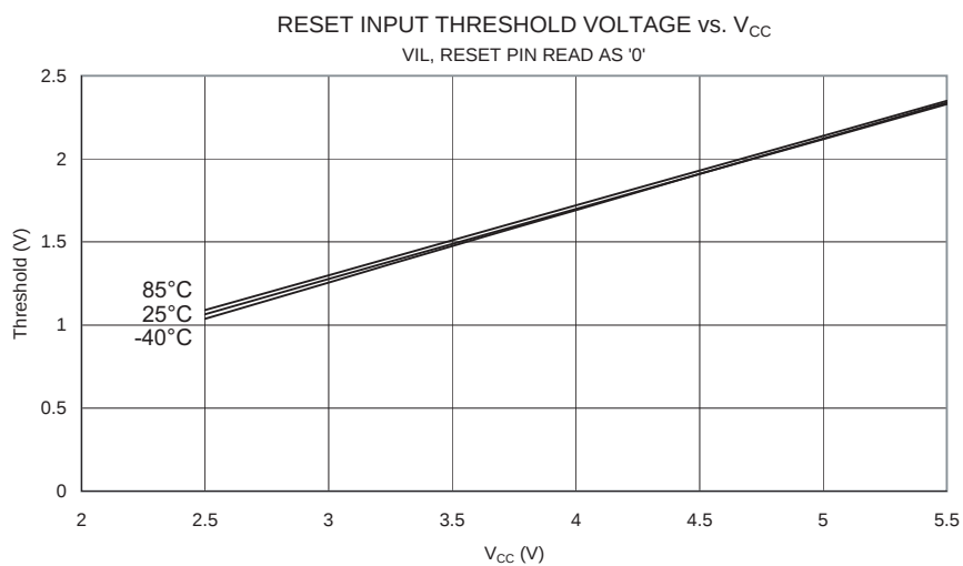
Figure 117. Reset 输入迟滞和 V_{CC} 的关系
