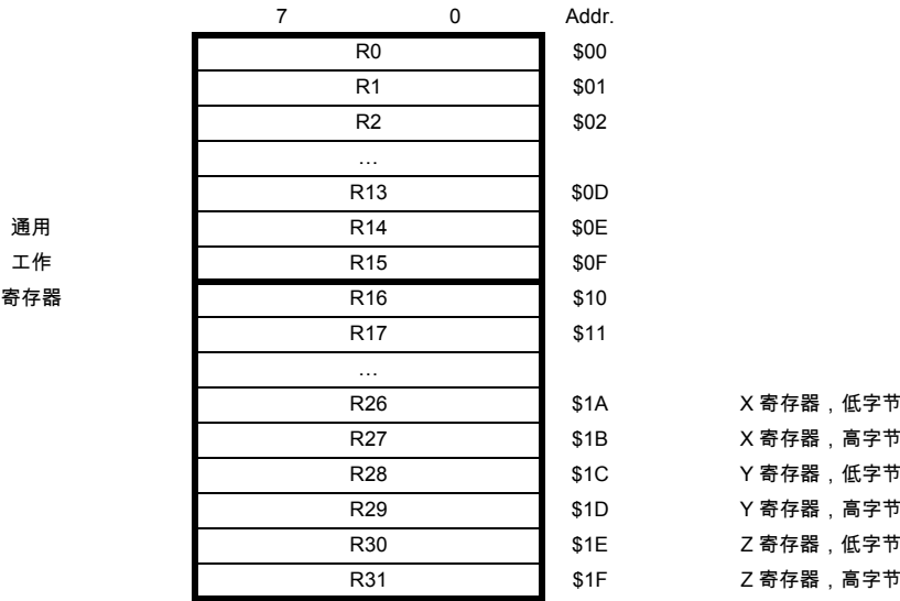
Figure 3. AVR CPU 通用工作寄存器
