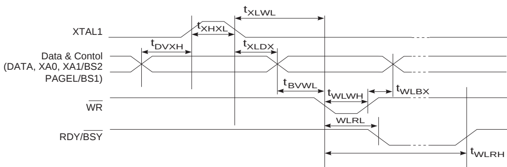
Figure 64. 并行编程时序, 包括一些常规的时序要求
