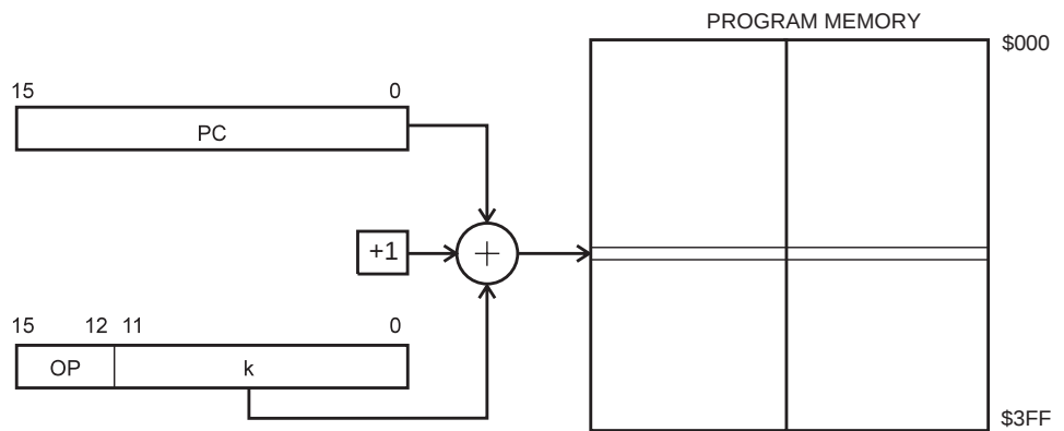
Figure 16. 相关程序存储器寻址
