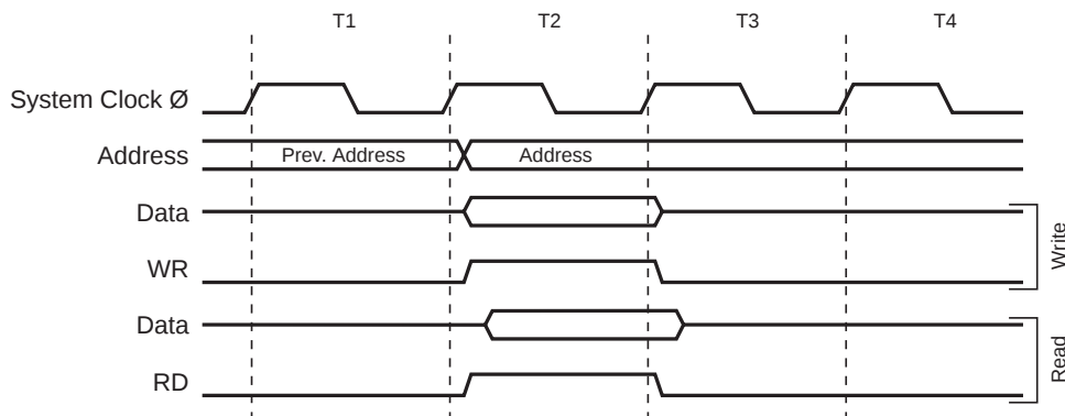
Figure 19. 片内数据 SRAM 访问周期
