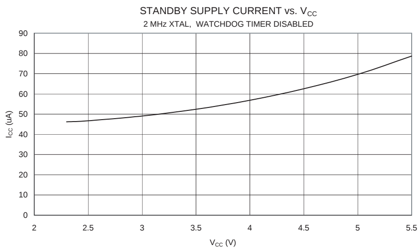
Figure 93. Standby 模式电流和 V_{CC} 的关系 (4 MHz 谐振器 , 看门狗定时器禁用 )
