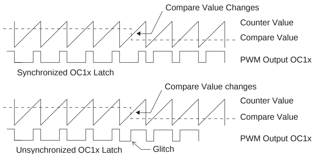
Figure 37. 非同步 OCR 锁存结果
