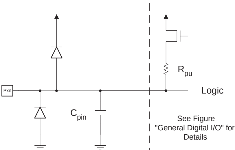
Figure 53. I/O 引脚等效原理图
