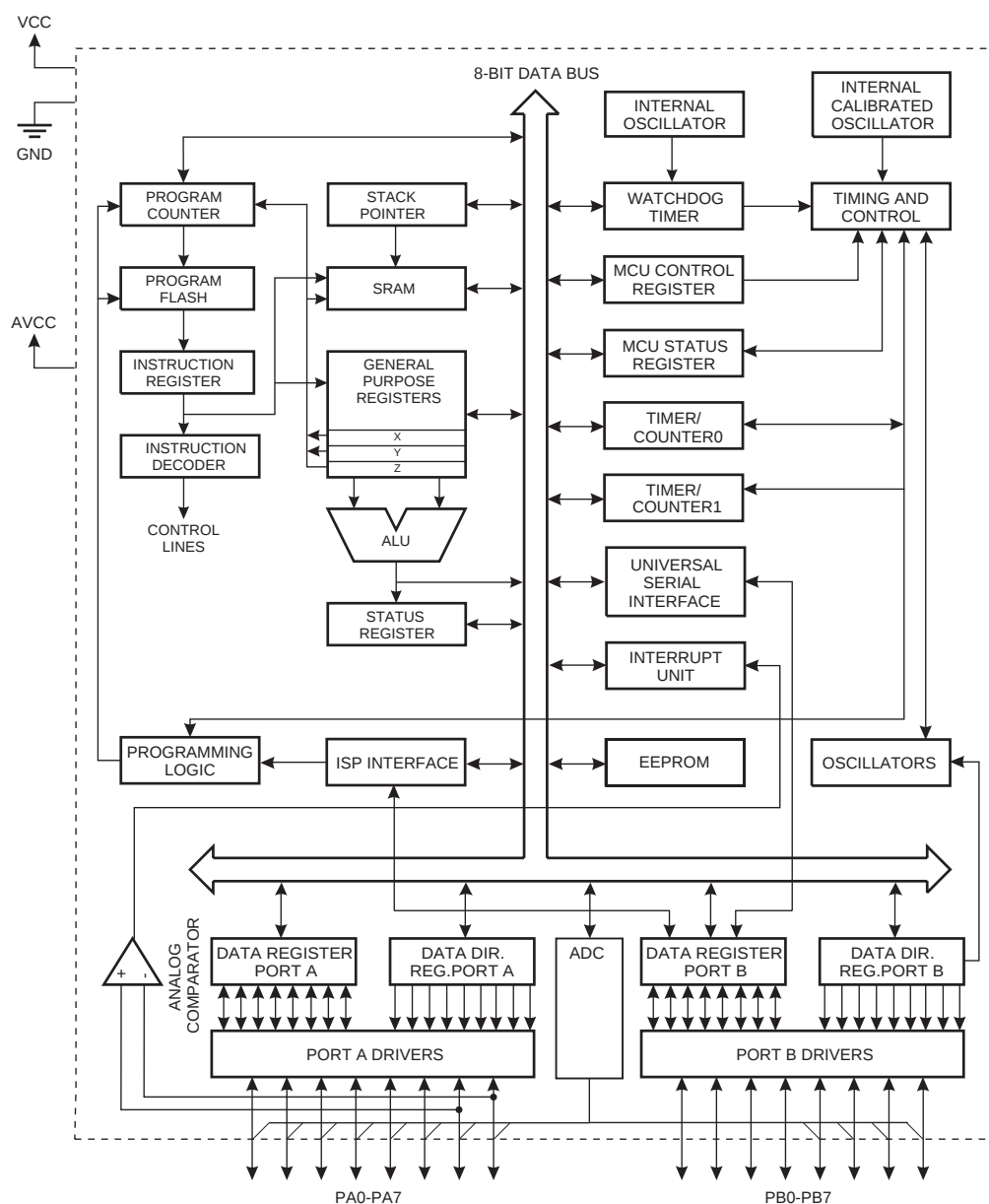
Figure 1. ATtiny26(L) 结构框图
