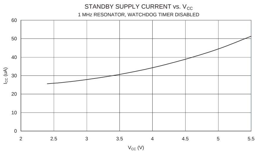
Figure 91. Standby 模式电流和 V_{CC} 的关系 (2 MHz 谐振器，看门狗定时器禁用)
