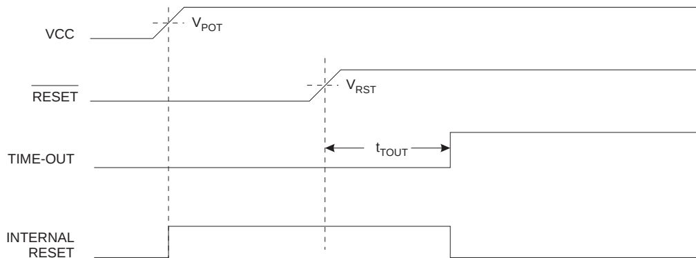
Figure 22. 外部控制 MCU 启动 RESET
