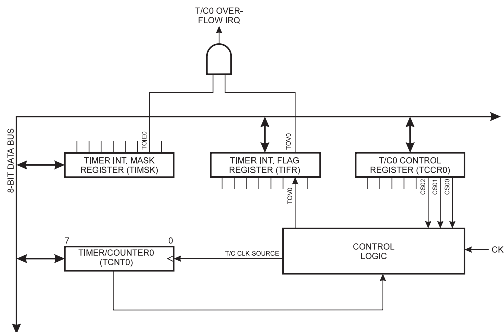
Figure 33. T/C0 方框图
