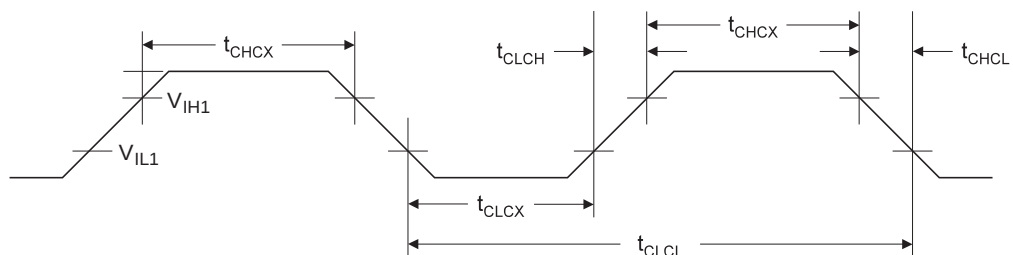
Figure 70. 外部时钟驱动波形
