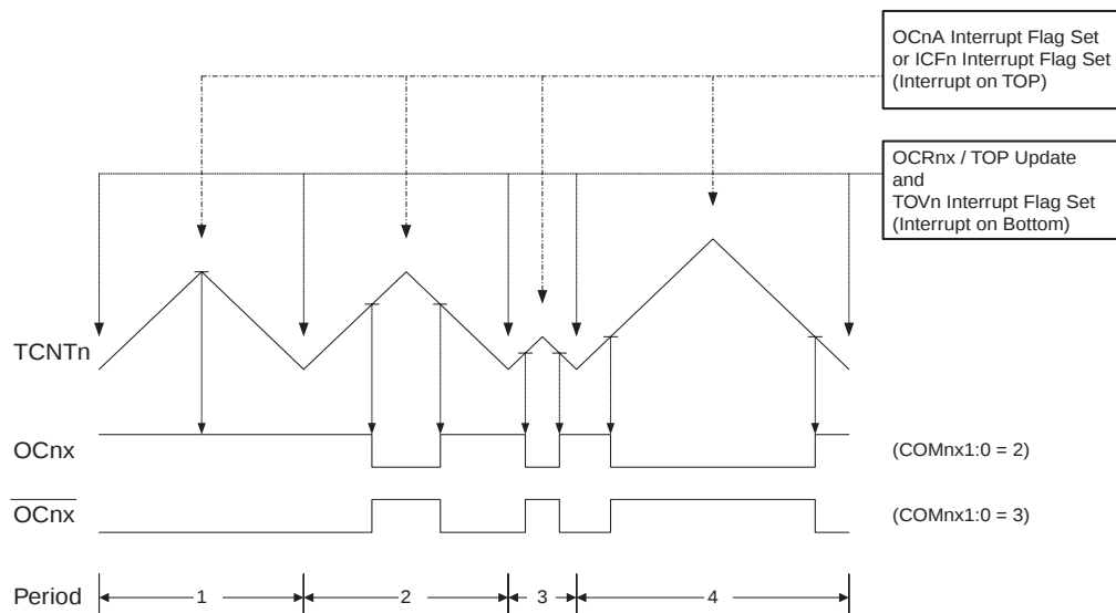
Figure 48. 相位与频率修正 PWM 模式的时序图
