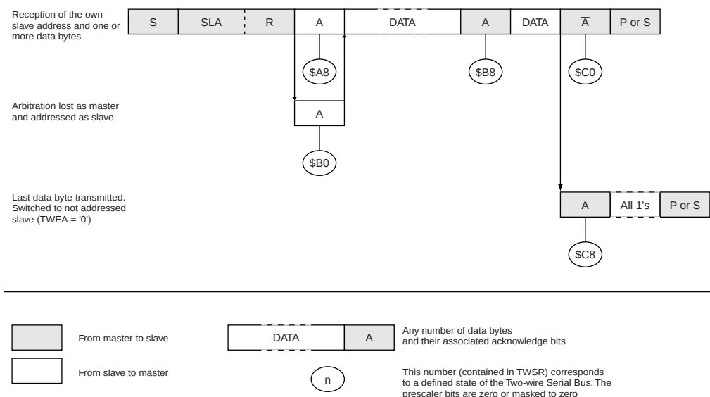
Figure 93. 从机发送模式的格式和状态
