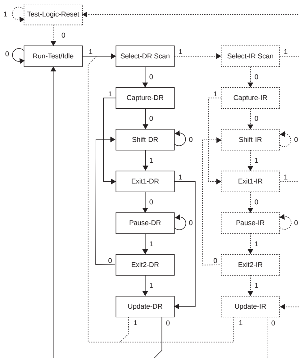
Figure 141. 改变 / 读取数据字的状态机序列
