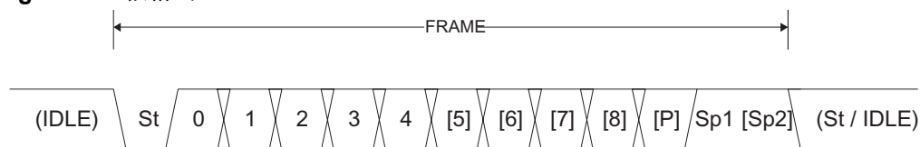
Figure 72. 帧格式
