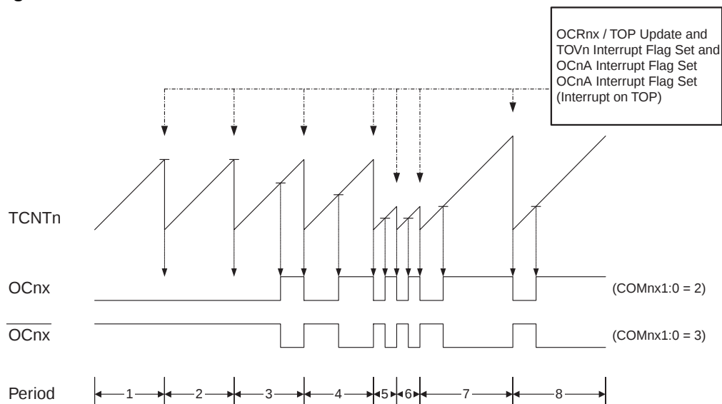
Figure 46. 快速 PWM 模式时序图
