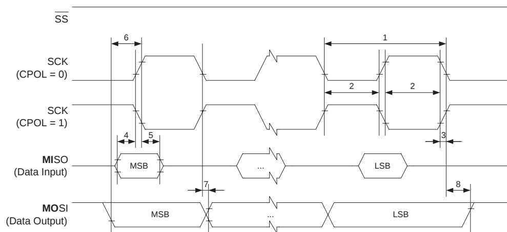
Figure 146. SPI 接口时序要求 (主机模式)
