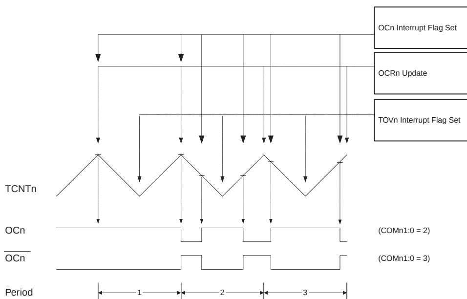
Figure 59. 相位修正 PWM 模式的时序图
