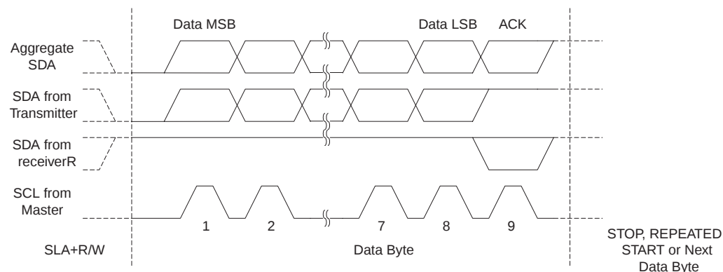
Figure 80. 数据包格式
