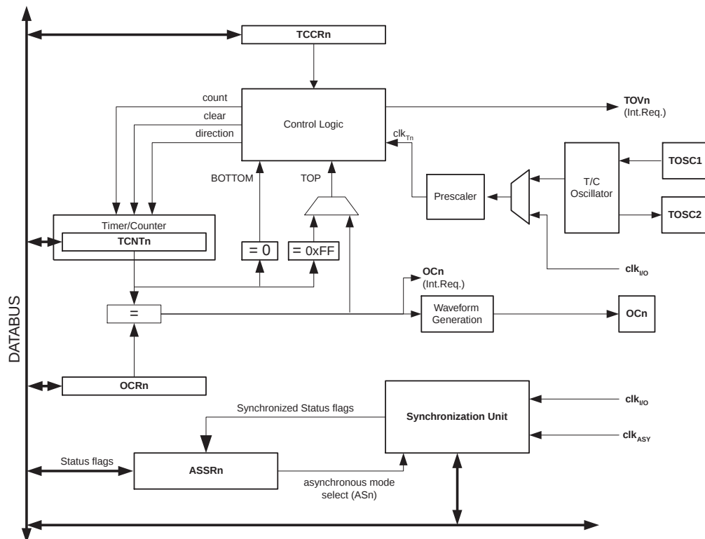
Figure 53. 8 位 T/C 方框图
