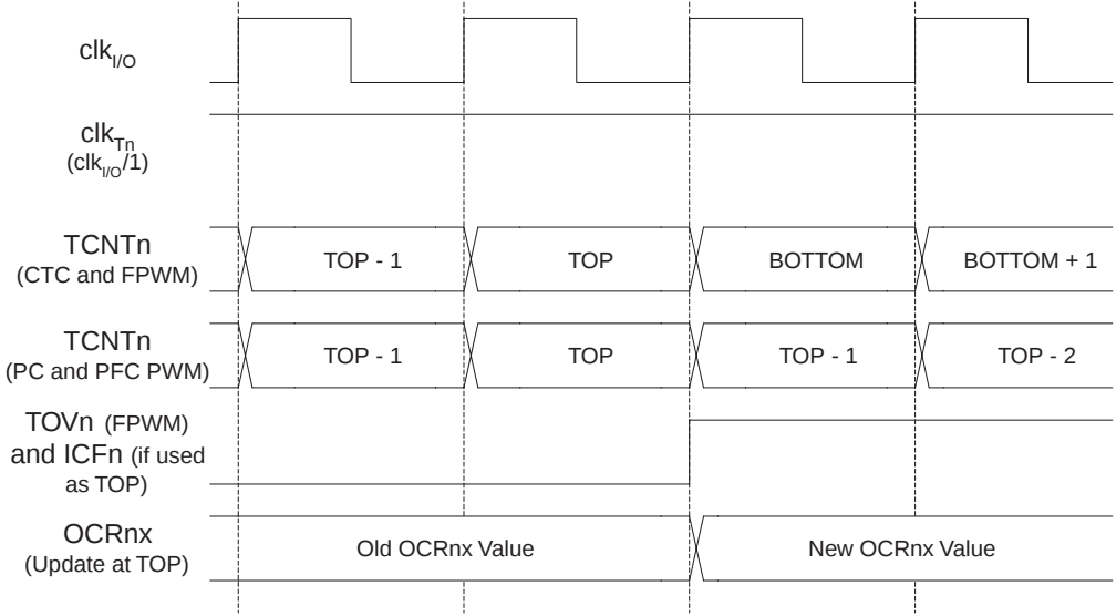
Figure 51. T/C 时序图，无预分频器
