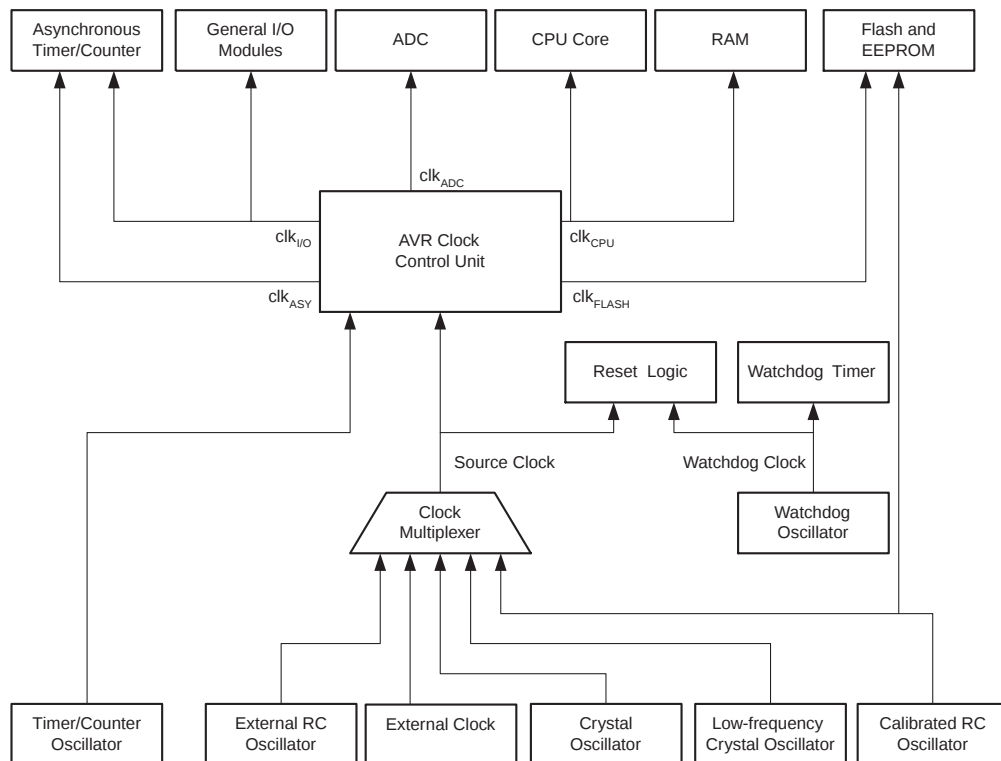
Figure 11. 时钟分布
