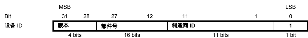
Figure 114. 器件识别寄存器的格式
