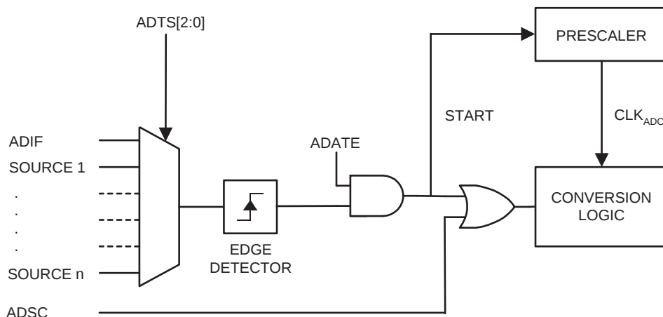
Figure 99. ADC 自动触发逻辑
