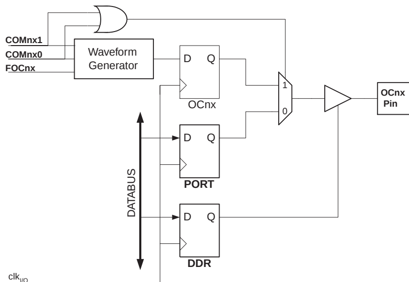
Figure 44. 比较匹配输出单元原理图
