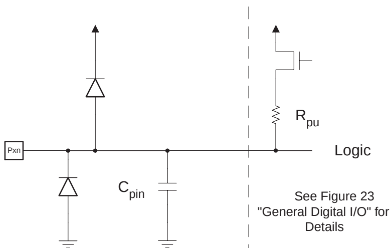
Figure 22. I/O 引脚等效原理图
