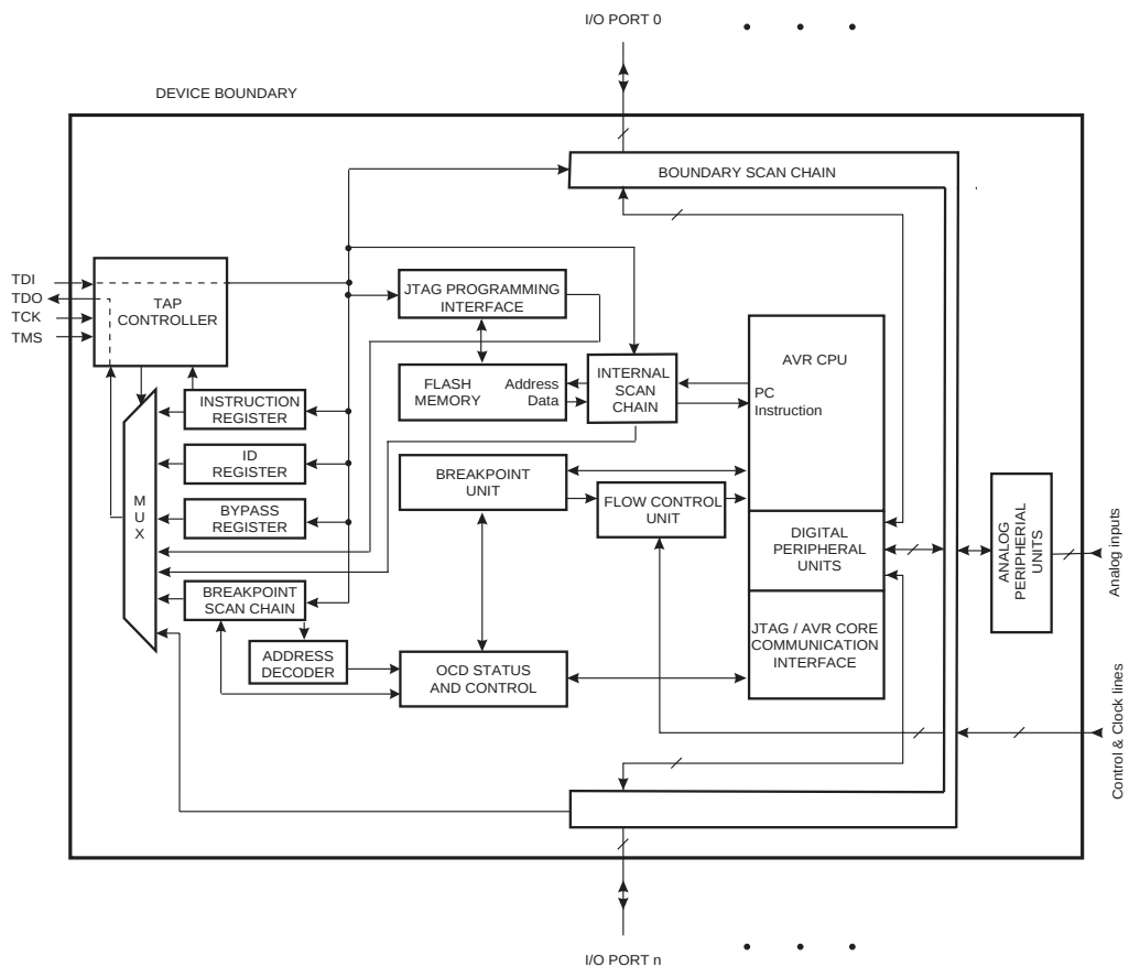
Figure 112. 方框图
