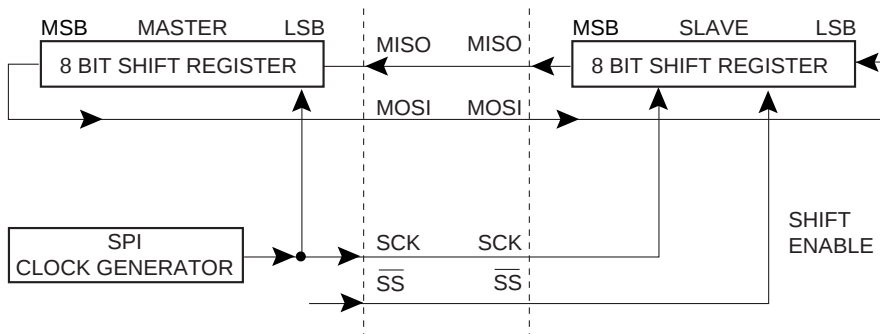
Figure 66. SPI 主机 - 从机的互连
