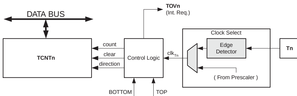
Figure 28. 计数器单元方框图
