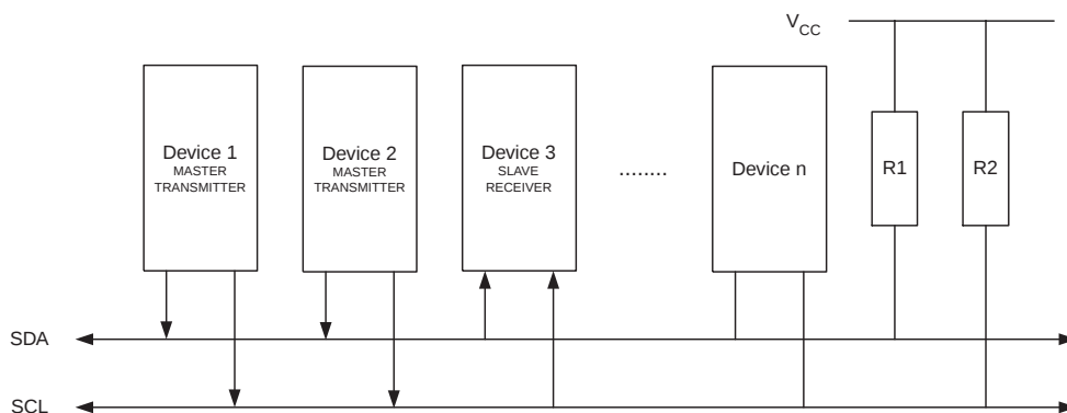
Figure 95. 仲裁示例
