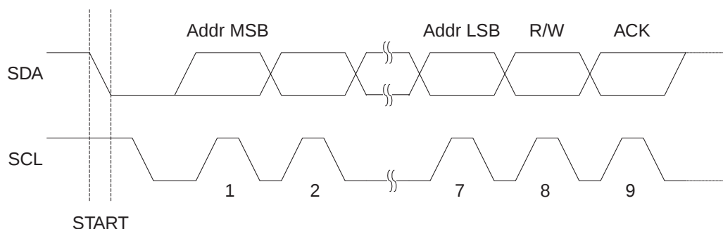
Figure 79. 地址包格式
