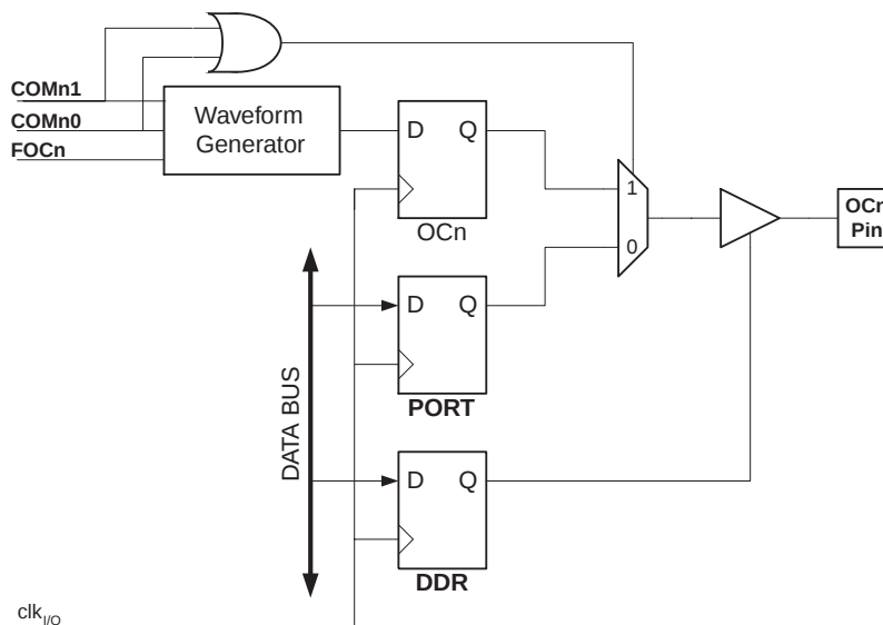
Figure 30. 比较匹配输出单元原理图
