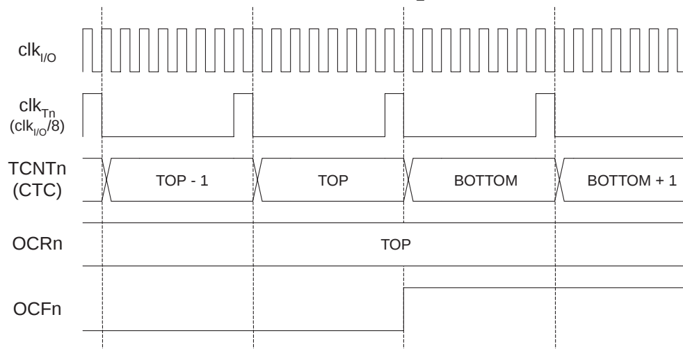
Figure 63. T/C 时序图，CTC 模式，预分频器为 f_{clk\_I/O}/8
