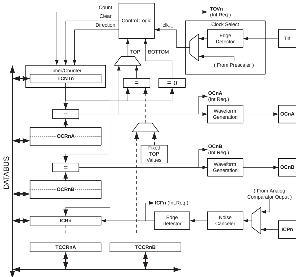
Figure 40. 16 位 T/C 框图 (1)
