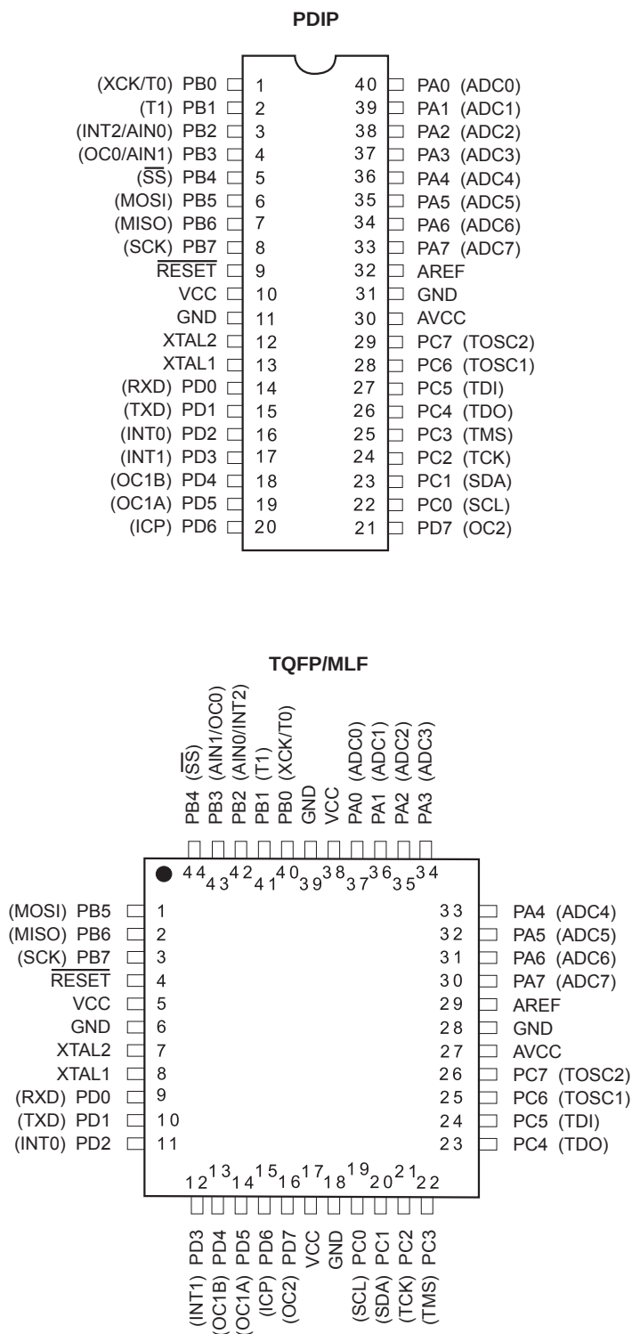
Figure 1. ATmega32 的引脚
