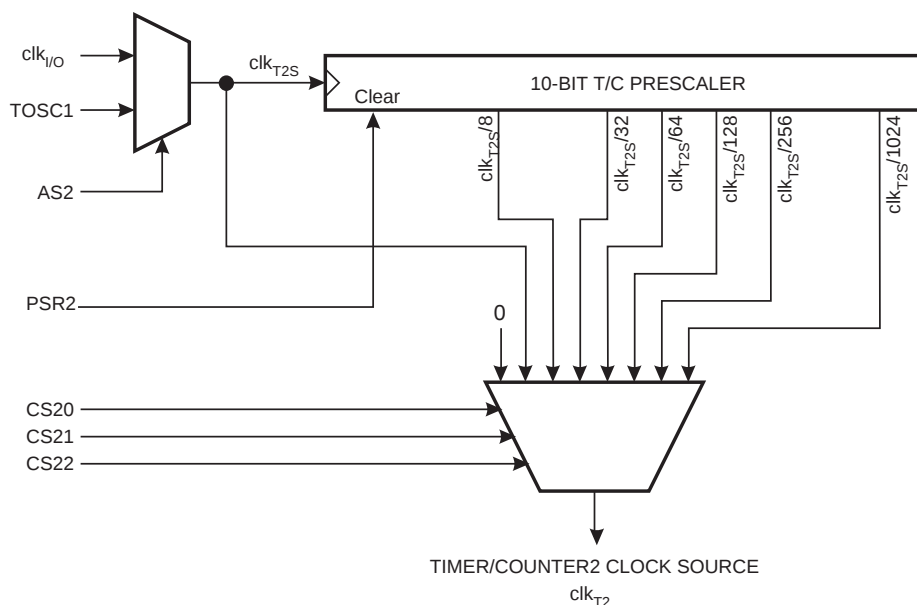
Figure 64. T/C2 的预分频器
