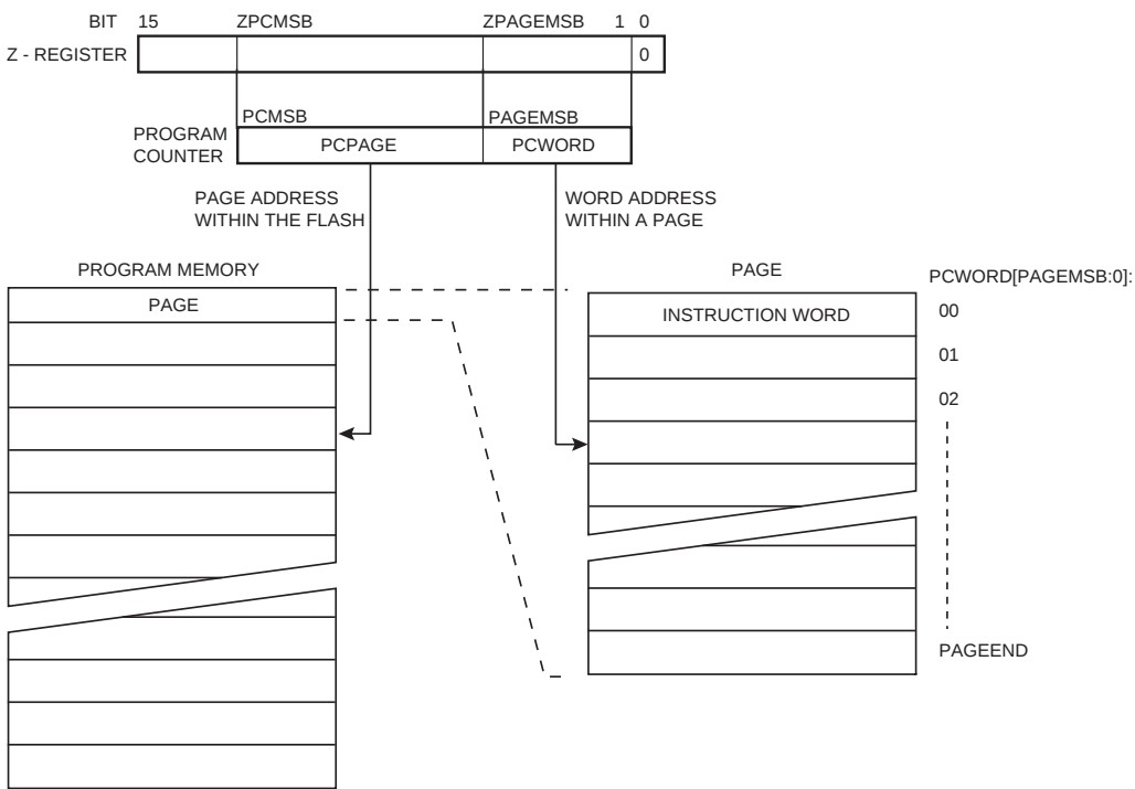
Figure 126. SPM 的寻址 (1)
