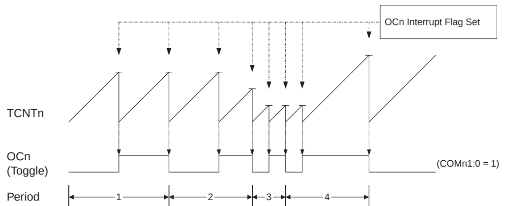
Figure 31. CTC 模式的时序图
