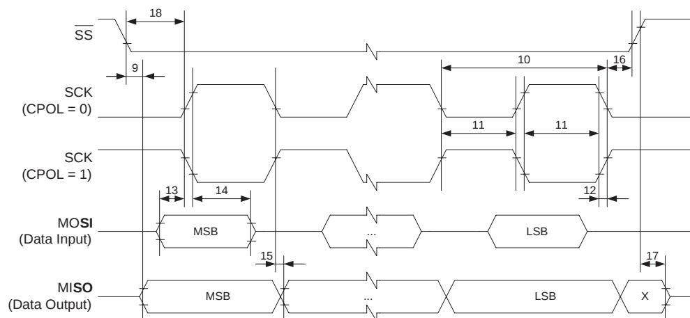
Figure 147. SPI 接口时序要求 (从机模式)
