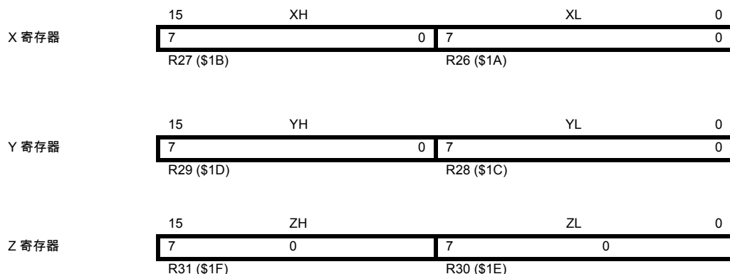
Figure 5. X、Y、Z 寄存器
