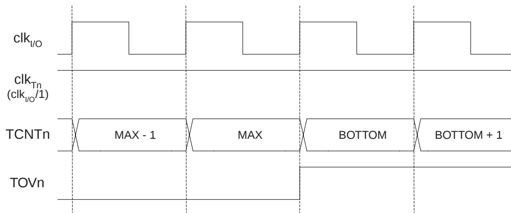
Figure 34. T/C 时序图，无预分频器
