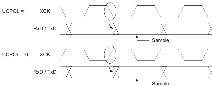
Figure 71. 同步模式时的 XCK 时序。
