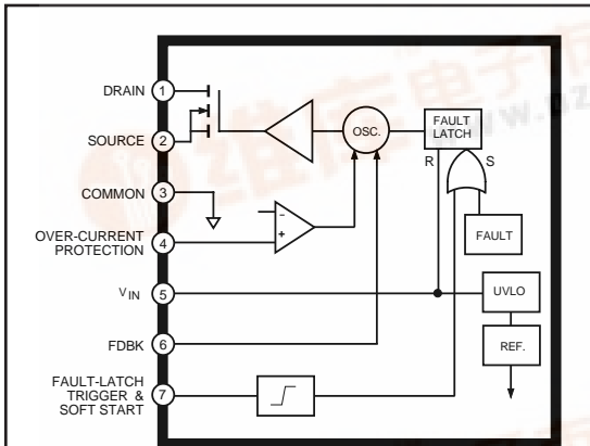
Dwg. PK-002
