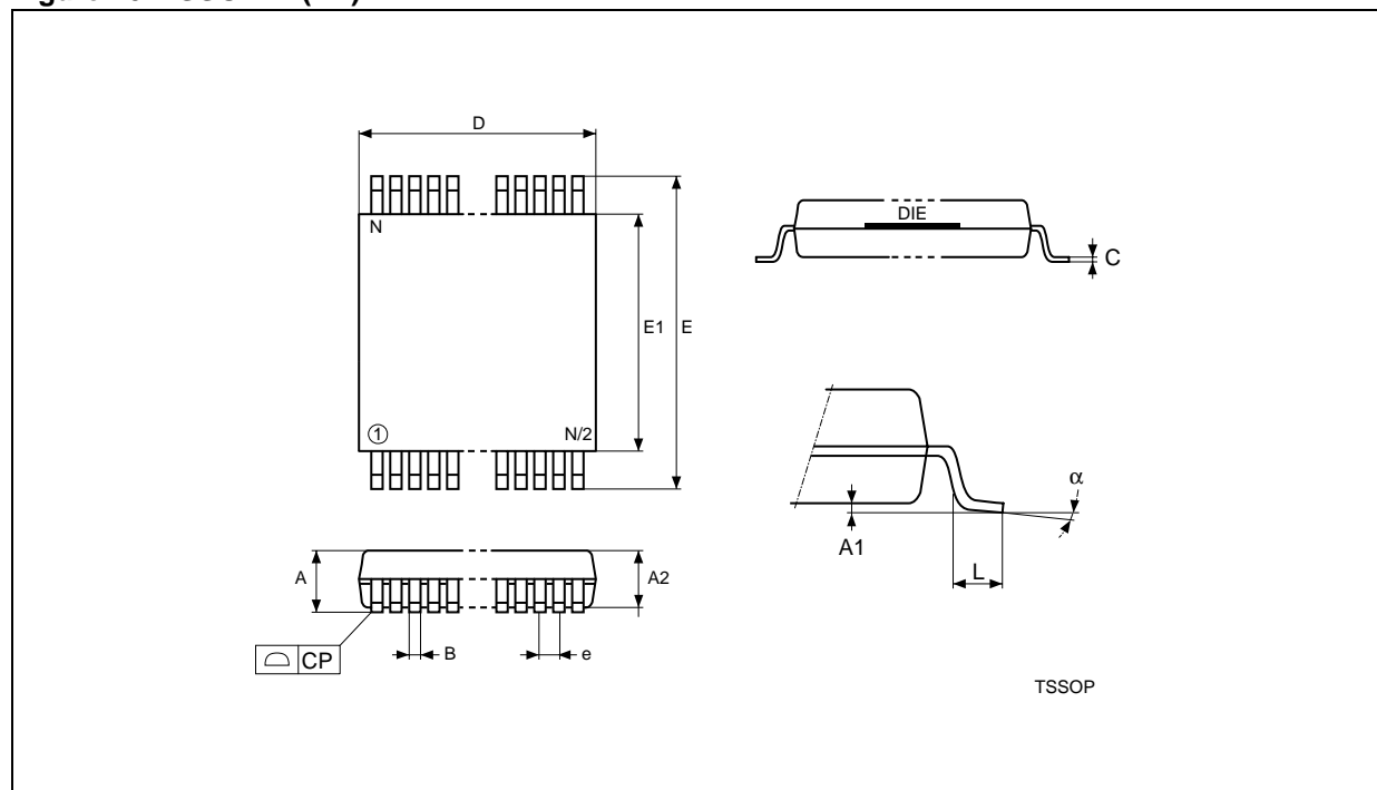
Figure 20. TSSOP14 (DL)
