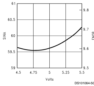
SINAD & ENOB vs V_A
