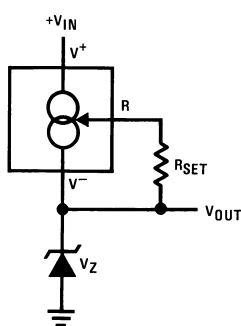
Zener Biasing
