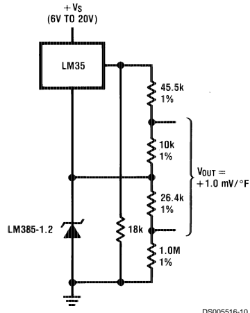
FIGURE 10. Fahrenheit Thermometer
