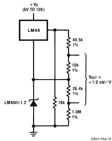
FIGURE 8. Fahrenheit Thermometer
