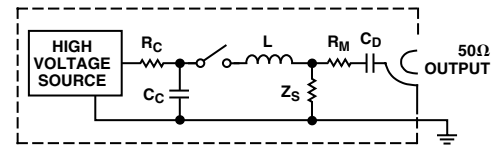
Figure 12. EFT Generator
