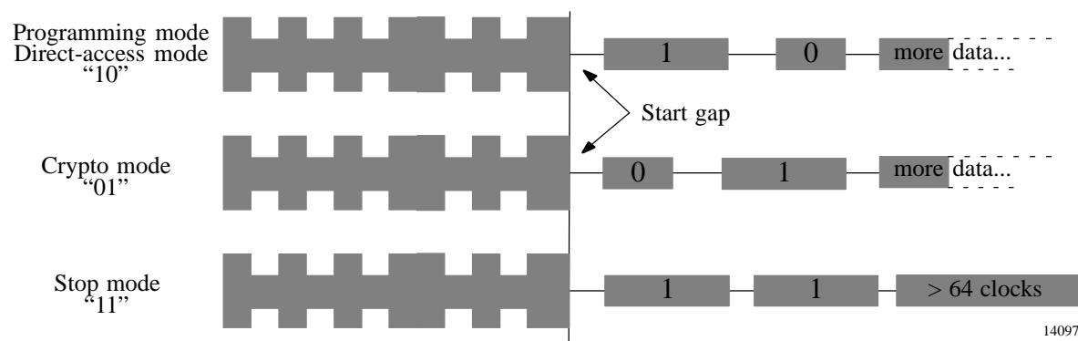
Figure 16. OP codes
