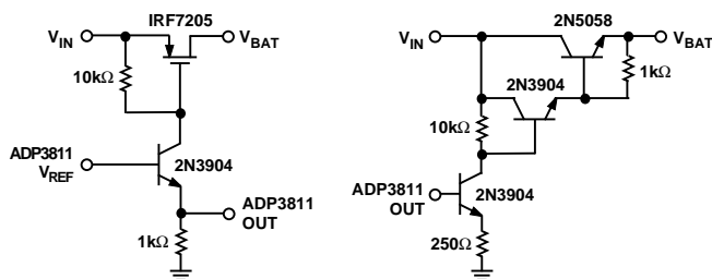
a. P-Channel MOSFET b. NPN Darlington
