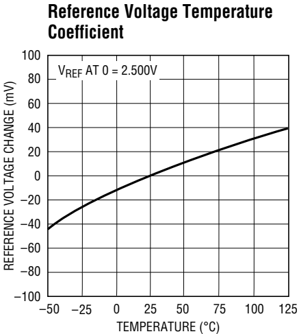
LT1054 • TPC10
