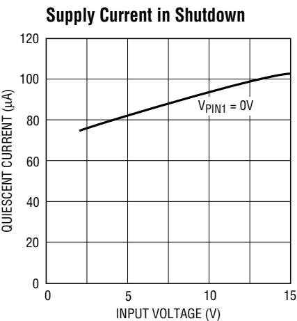
LT1054 • TPC04
