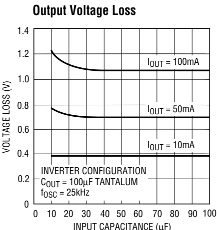
LT1054 • TPC06
