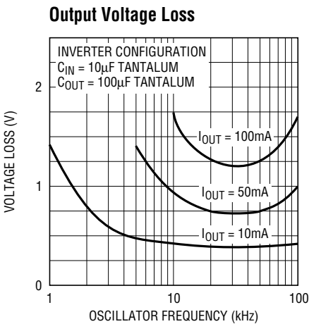
LT1054 • TPC07
