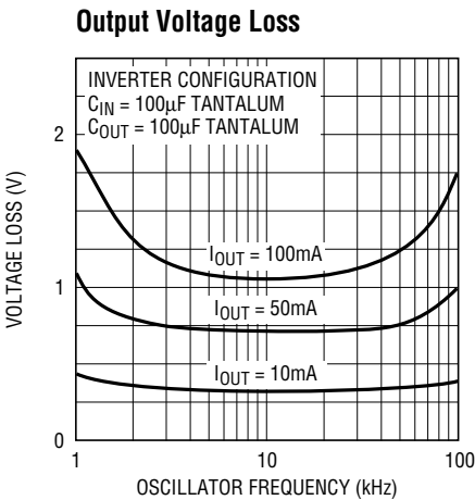
LT1054 • TPC08
