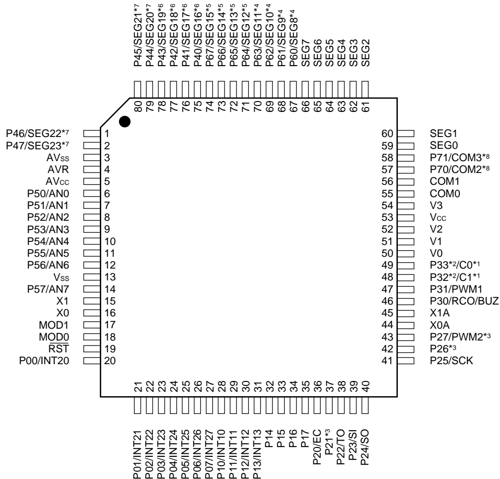
(FPT-80P-M05)
