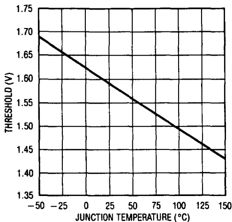
Enable Threshold
