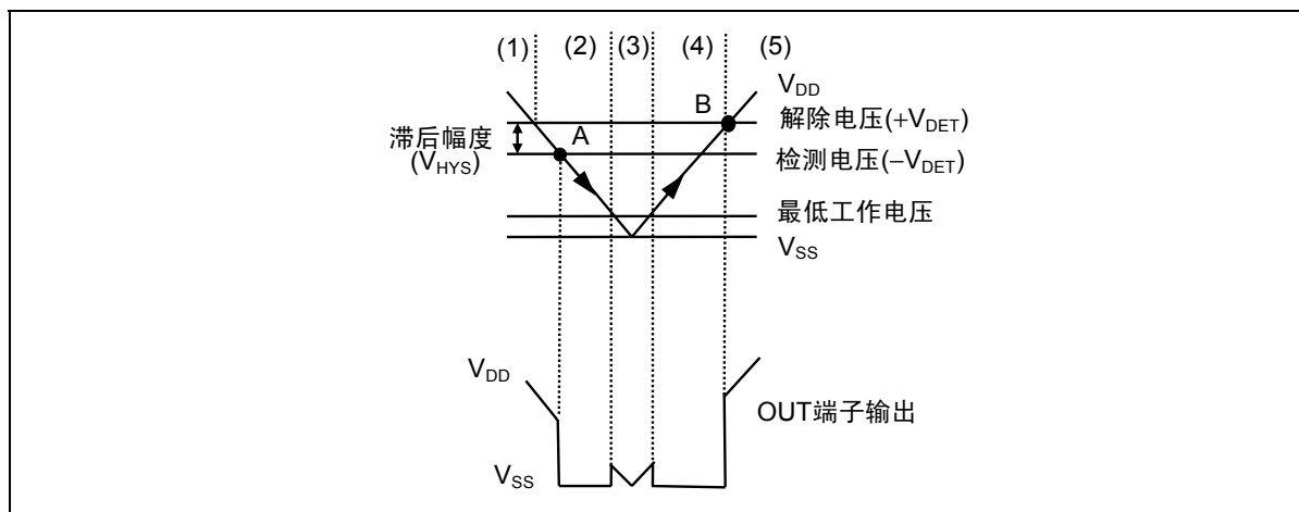
图16 工作说明图2
