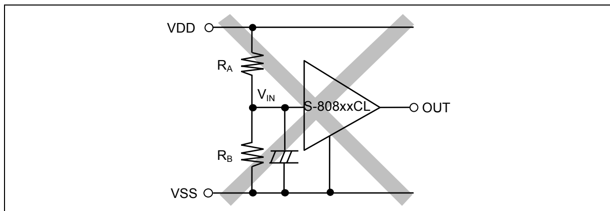
图21 检测电压改变电路不良事例
