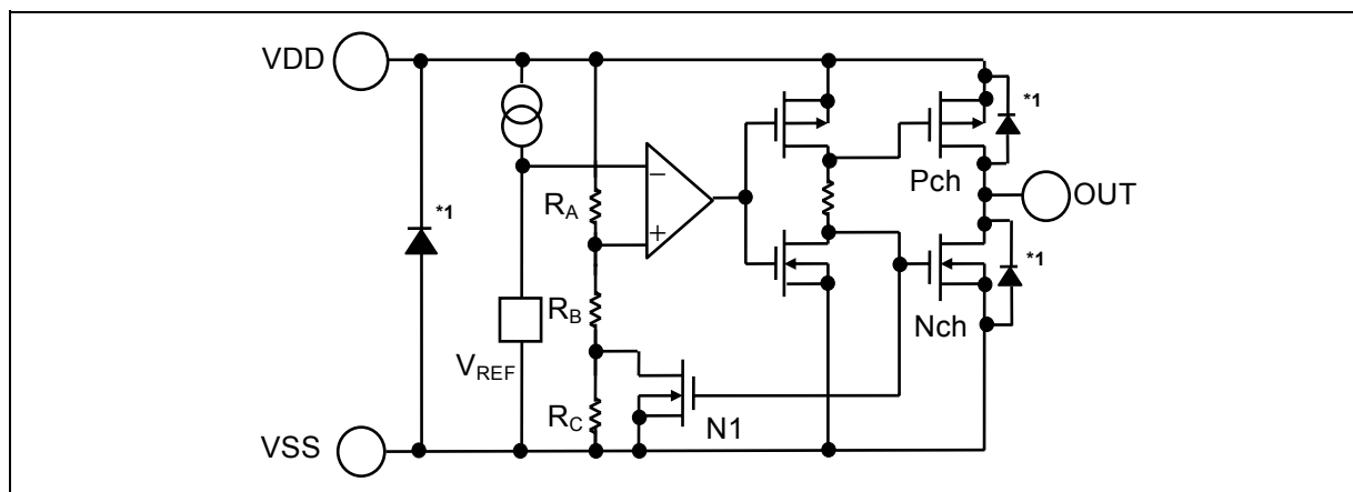
图15 工作说明图1
