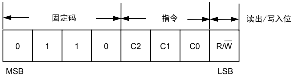
图9 通信数据
