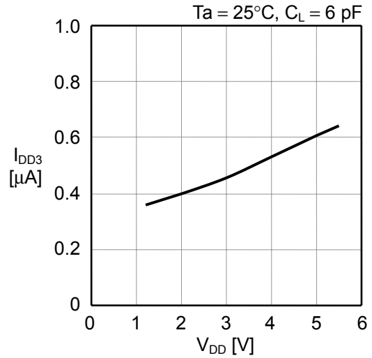
(2) 32 kHz输出时消耗电流 - V_{DD} 特性
