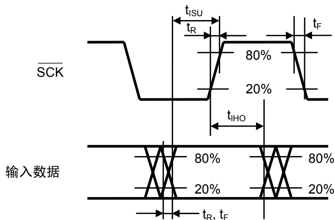
图7 AC特性2
