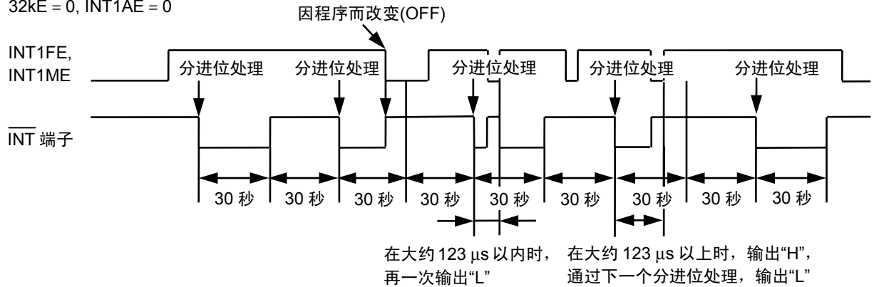
图22 分单位稳态中断输出1时序
