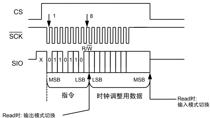
图30 时钟调整用寄存器存取
