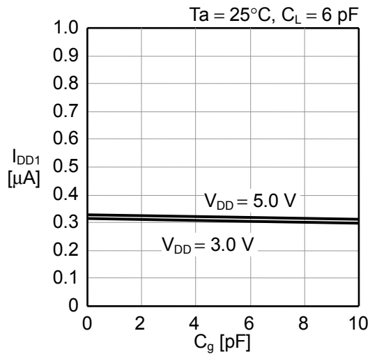
(5) 待机电流 - C_g 特性
