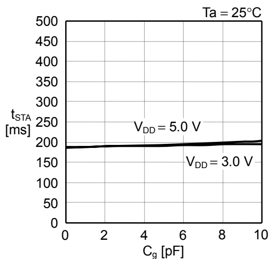
(9) 振荡开始时间 - C_g 特性
