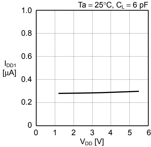
(1) 待机电流 - V_{DD} 特性
