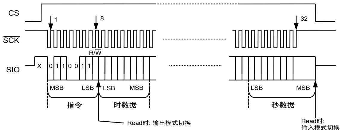
图26 实时数据存取2
