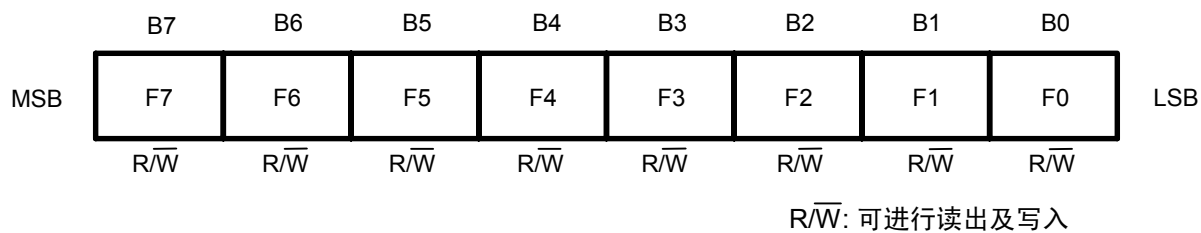
图17 自由寄存器
