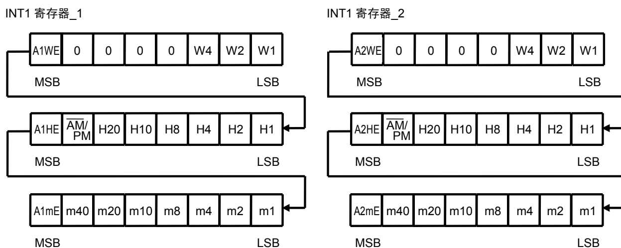
图13 INT1寄存器_1、INT1寄存器_2 (报警时刻数据)
