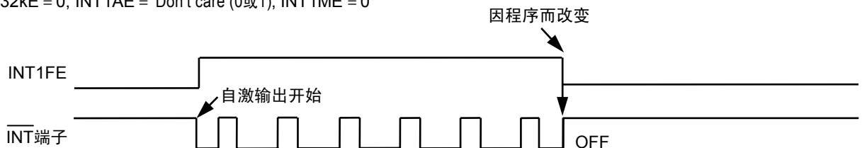
图20 选择频率稳态中断输出时序
