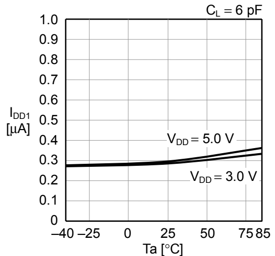
(4) 待机电流 - 温度特性
