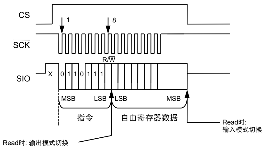
图31 自由寄存器存取
