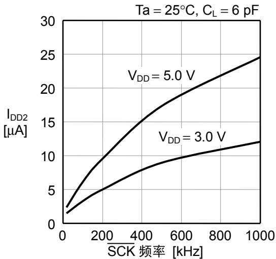
(3) 工作时消耗电流 - 输入时钟特性
