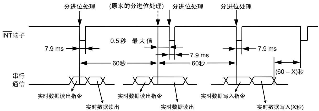
图23 分单位稳态中断输出2时序
