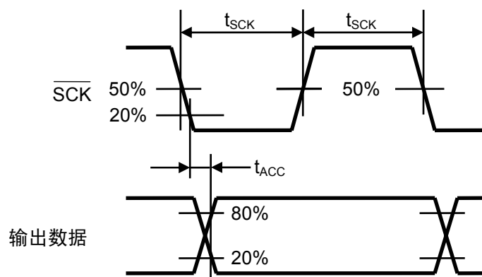
图8 AC特性3
