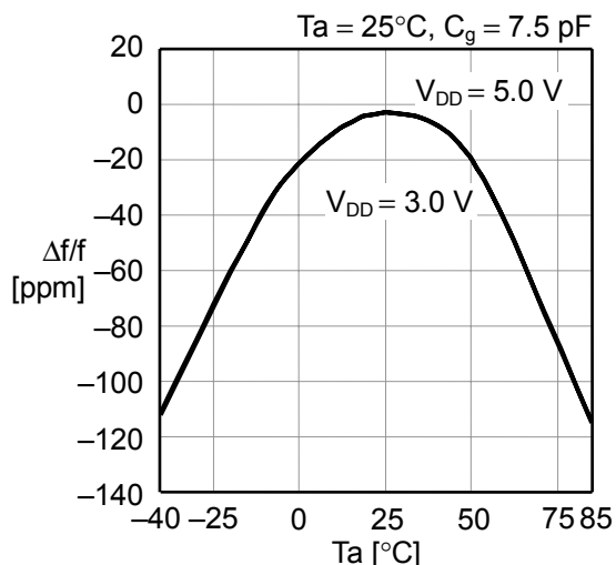
(8) 振荡频率 - 温度特性
