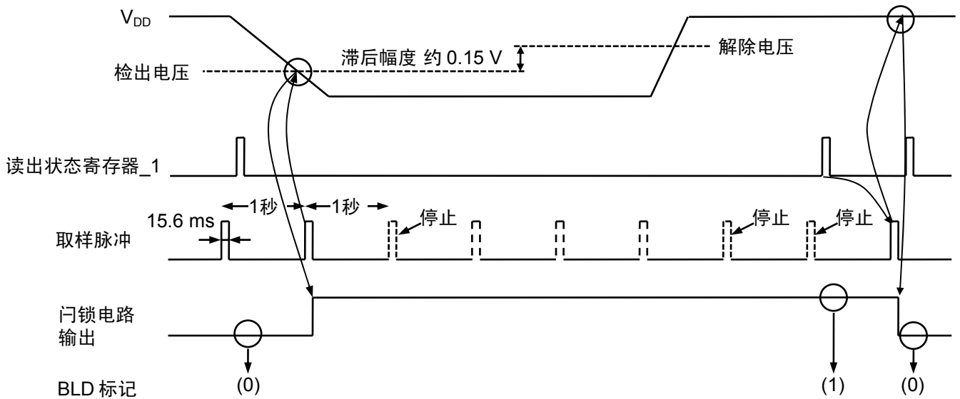
图18 电源电压检测电路时序
