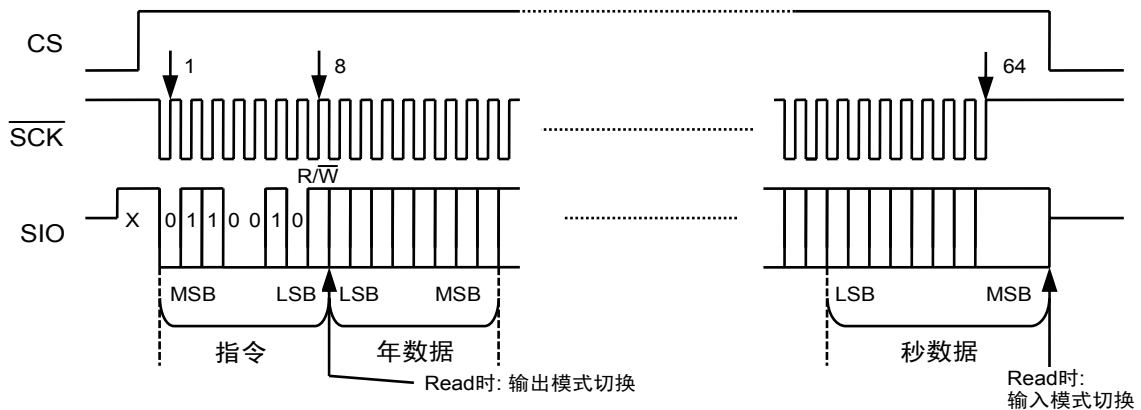
图25 实时数据存取1
