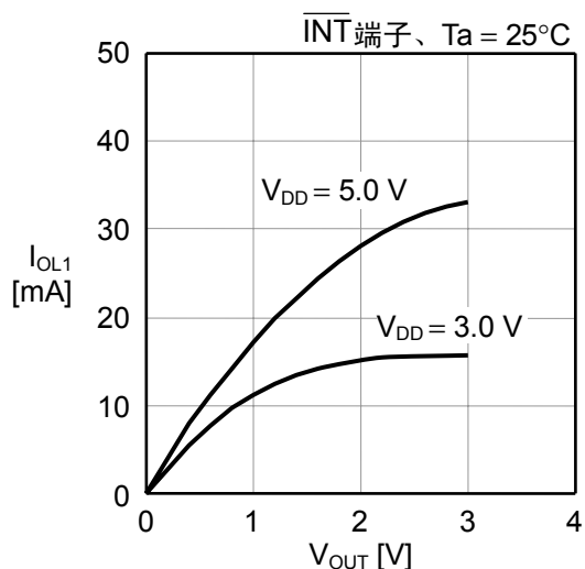
(10) 输出电流特性1 ( V_{OUT} - I_{OL1} )
