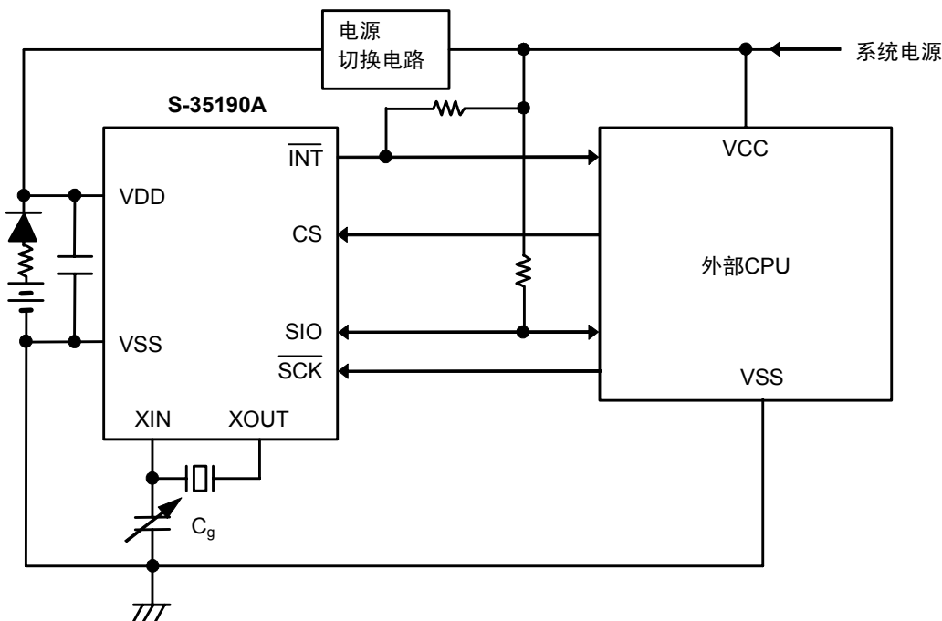
图33 应用电路1
