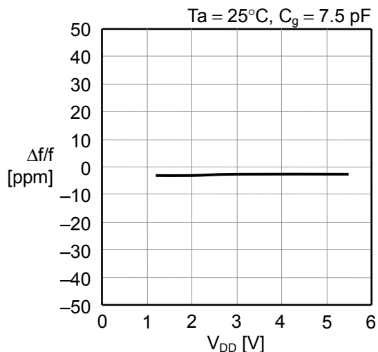
(7) 振荡频率 - V_{DD} 特性
