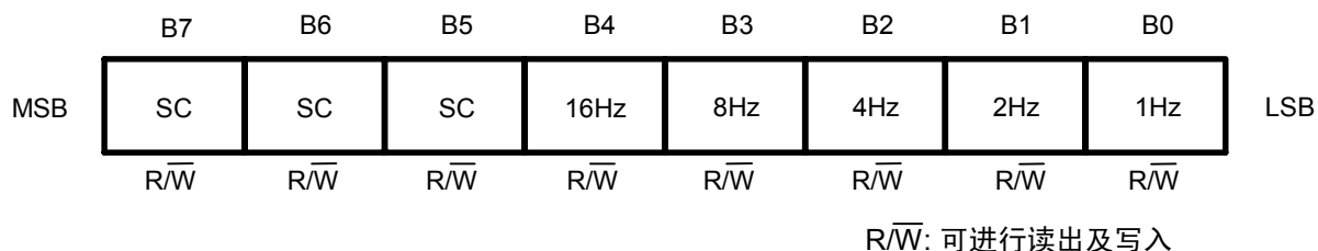
图14 INT1寄存器_1 (频率占空系数数据)
