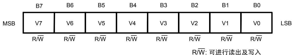
图16 时钟调整用寄存器
