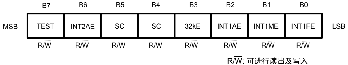
图12 状态寄存器_2
