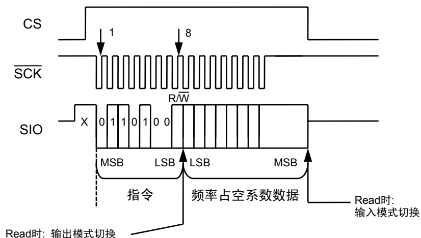
图29 INT1寄存器_1 (频率占空系数数据) 存取
