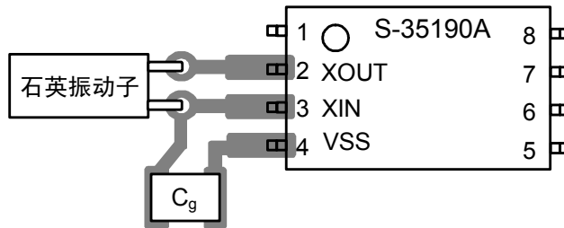
图36 连接图2
