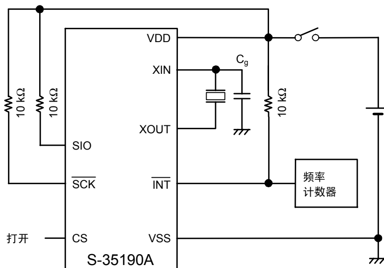
图37 振荡频率的测定电路构成
