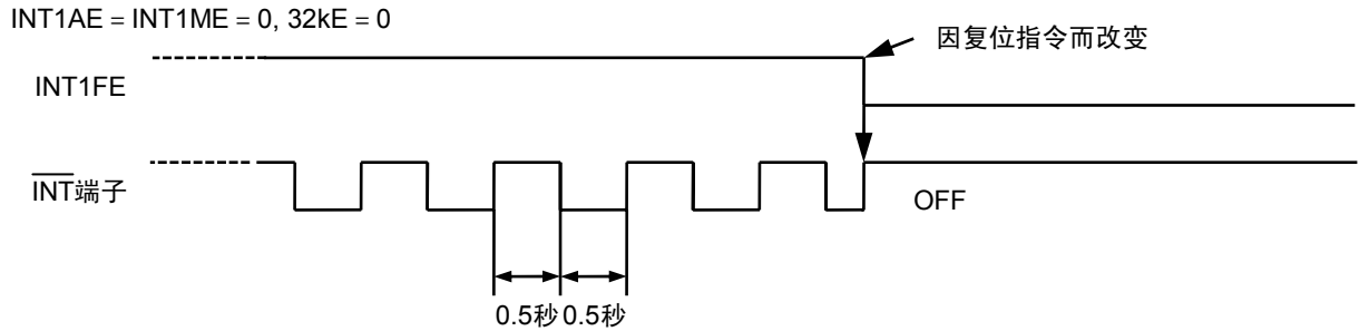
图24 电源接通检测电路工作时的 \overline{\text{INT}} 端子输出时序
