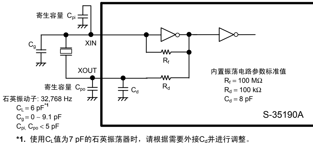
图35 连接图1
