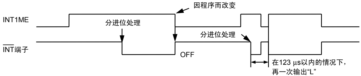
图21 分单位边缘中断输出时序
