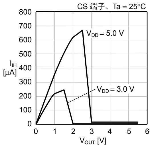
(12) CS端子输入电流特性
