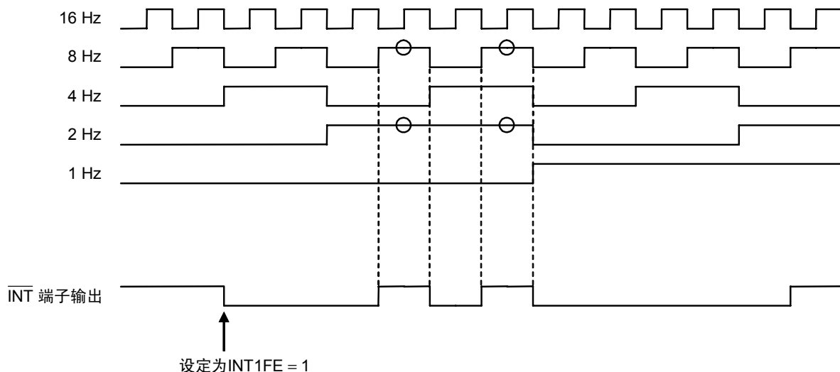
图15 INT1寄存器_1 (频率占空系数数据)的输出例
