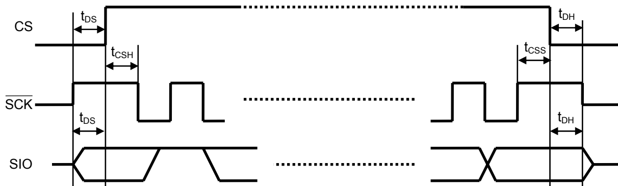
图6 AC特性1
