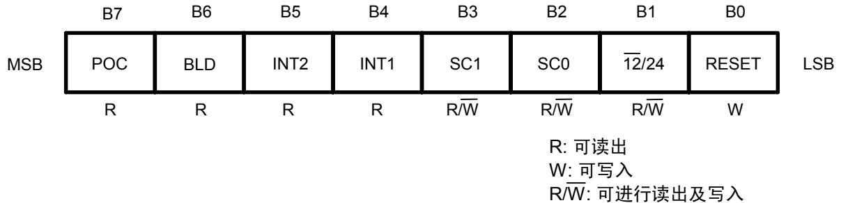
图11 状态寄存器_1
