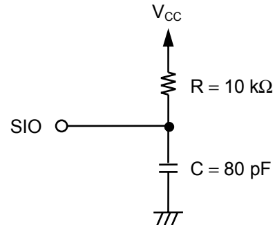
图5 输出负载电路
