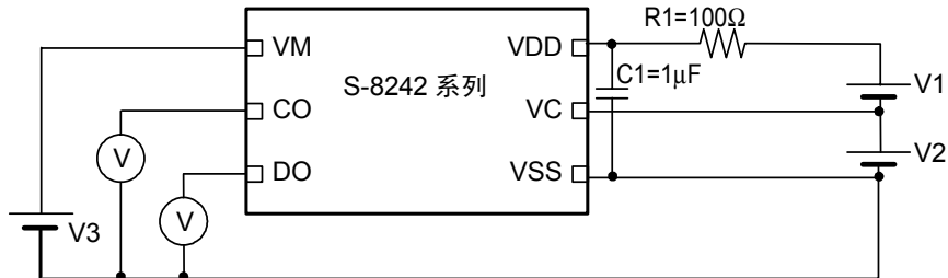
图4 测定电路1
