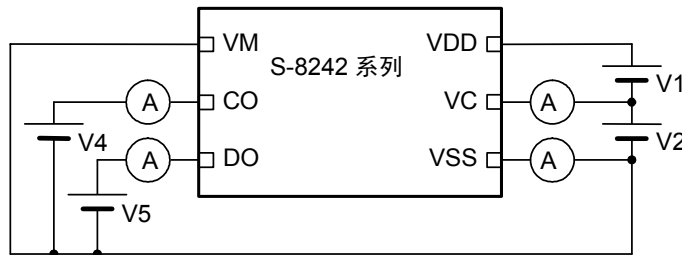
图7 测定电路4
