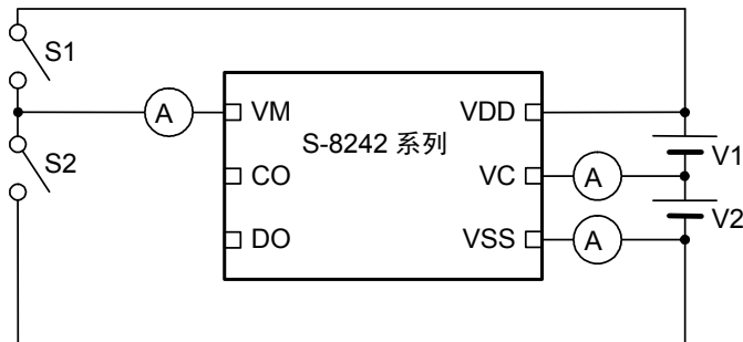
图6 测定电路3
