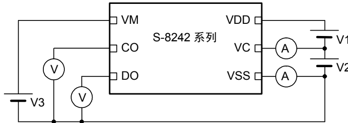
图5 测定电路2
