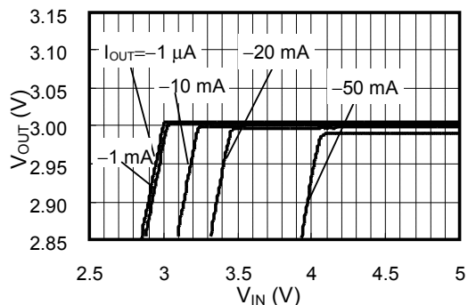
S-812C30B( T_a=25^\circ\text{C} )
