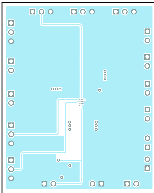
Figure 21. EVM Layer 2
