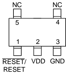
SOT-23-5
