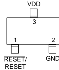
SOT-23-3
