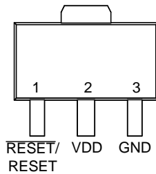
SOT-89
