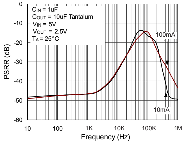
PSRR
