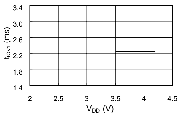
过电流2检测延迟时间—电源电压特性
