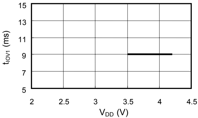
过电流1检测延迟时间—电源电压特性
