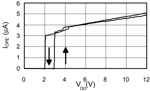
消耗电流—电源电压特性
