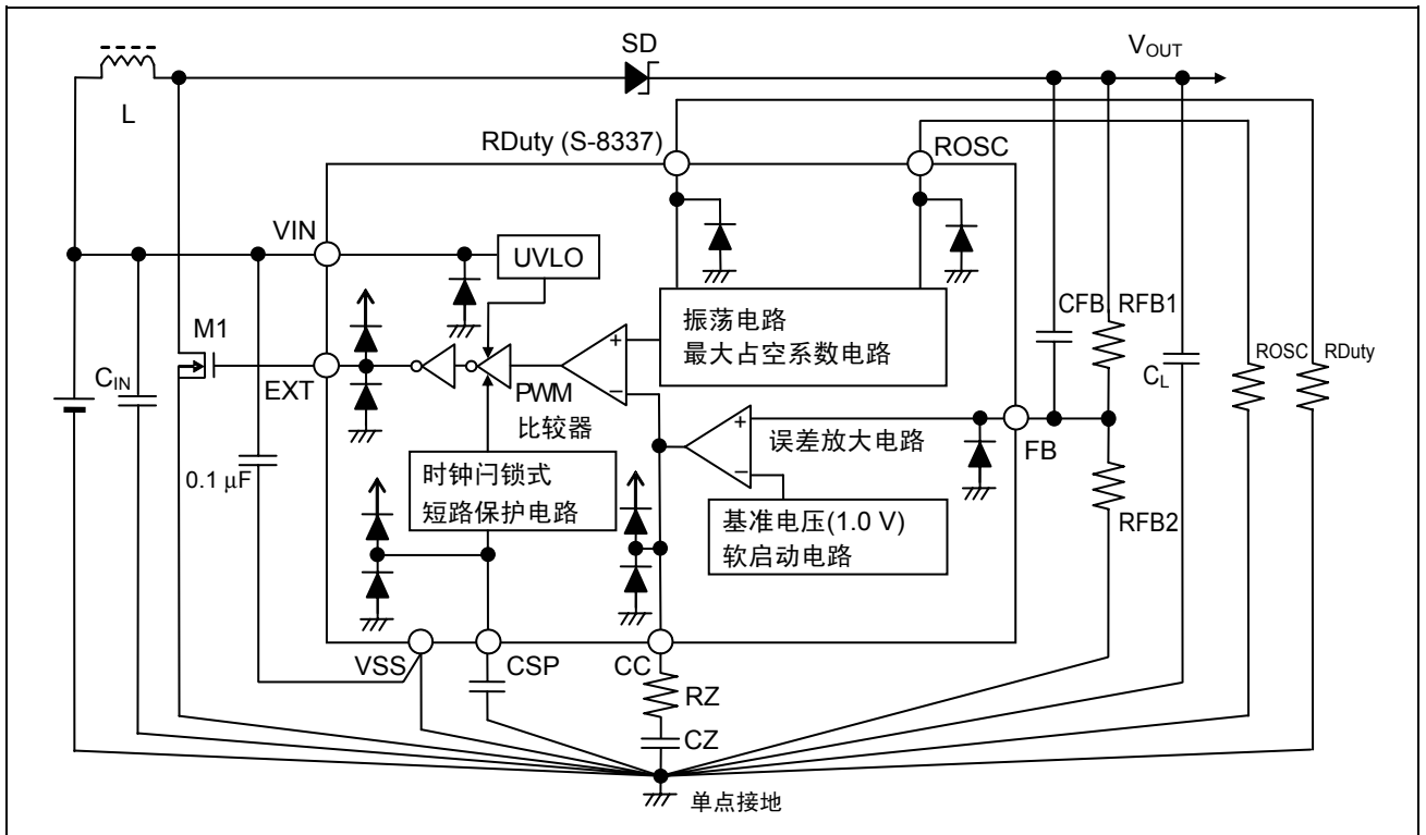
图 14 标准电路 (S-8337 系列)
