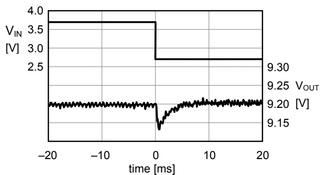
4-6. f_{OSC} = 286\text{ kHz} , V_{IN} = 3.7\text{ V} \rightarrow 2.7\text{ V}
