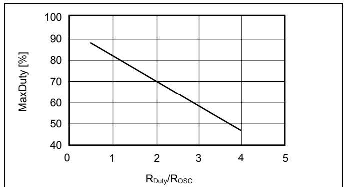
图 12 R Duty /R OSC vs. MaxDuty
