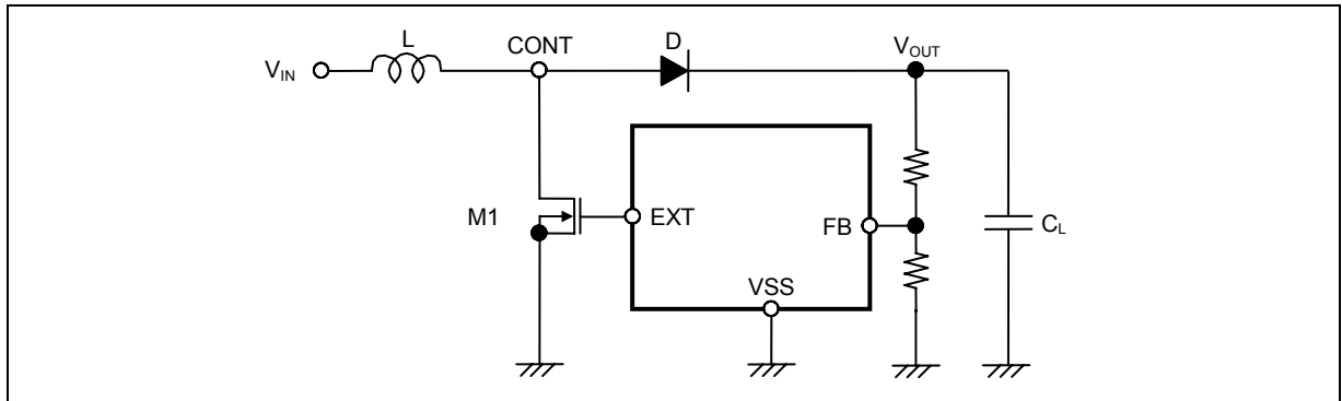
图 9 升压型 DC/DC 控制器的基本方式电路
