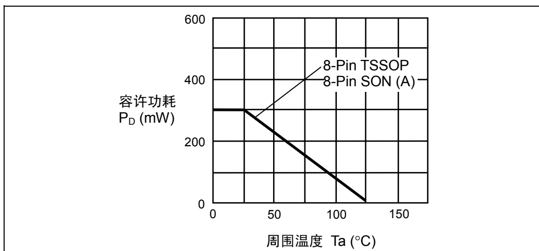
图 16 封装容许功耗(未安装时)
