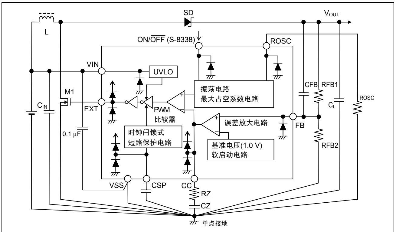
图 15 标准电路 (S-8338 系列)
