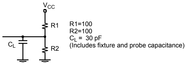
TTL AC Test Load
