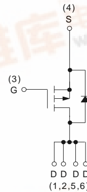
P-Channel MOSFET
