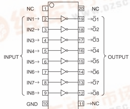
20P2N-A(FP)
