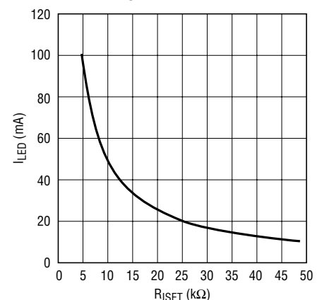
I_{LED} vs R_{ISET}
