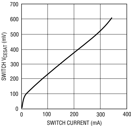
Switch V_{CESAT}
