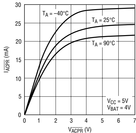
ACPR Pin I-V Curve (Pull-Down State)
