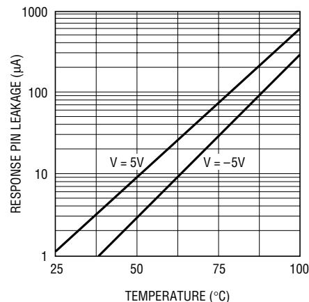
LT1032 • G06
