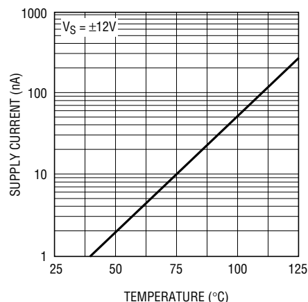
LT1032 • TPC03
