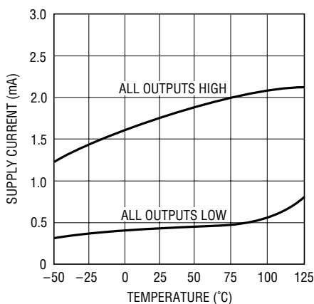
LT1032 • TPC01
