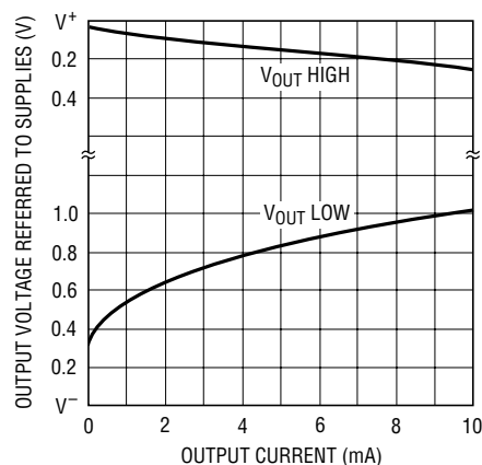
LT1032 • TA02
