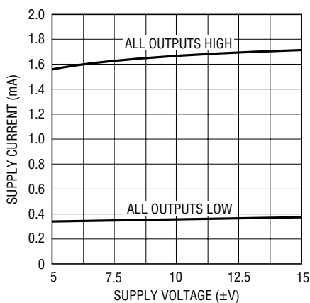
LT1032 • TPC02
