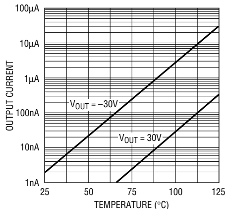
LT1032 • TPC05
