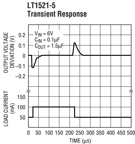
LT1521 • TPC33
