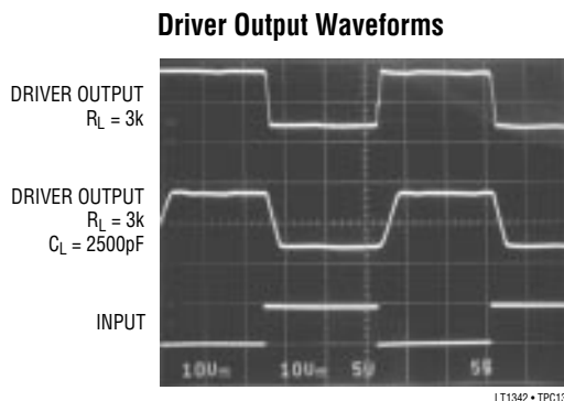
LT1342 • TPC13
