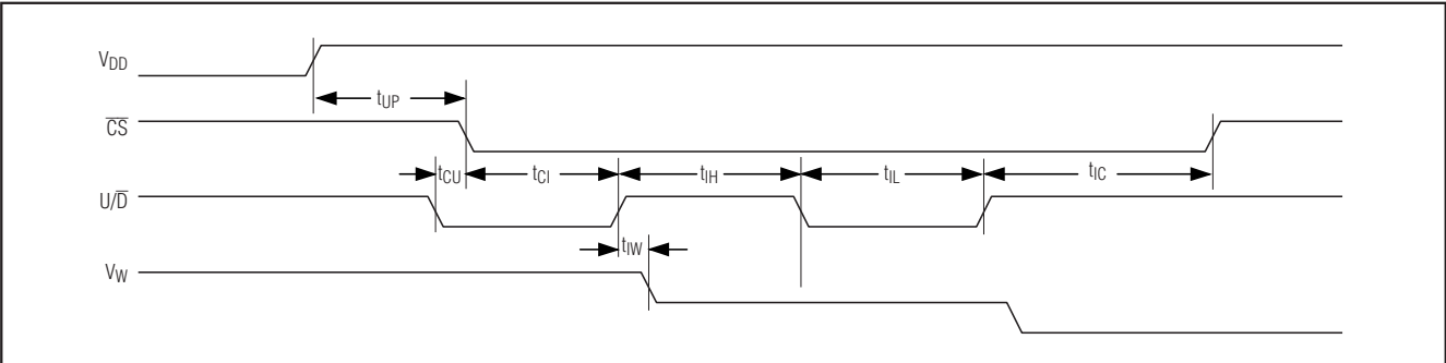
图3. 递减模式时序图
