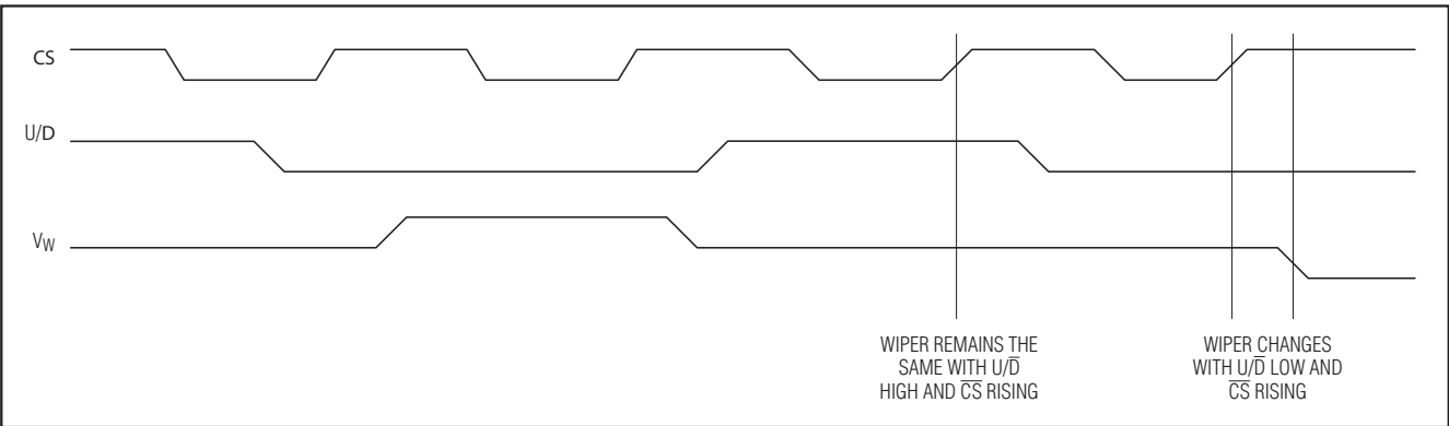
图4. CS由低电平至高电平跳变的时序图
