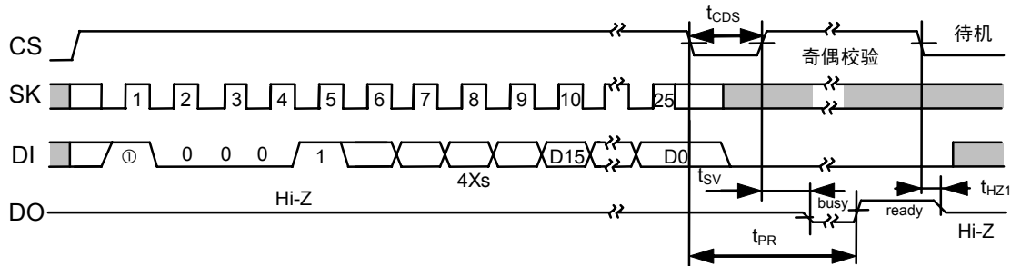
图13 全部写入定时(S-93L46A)
