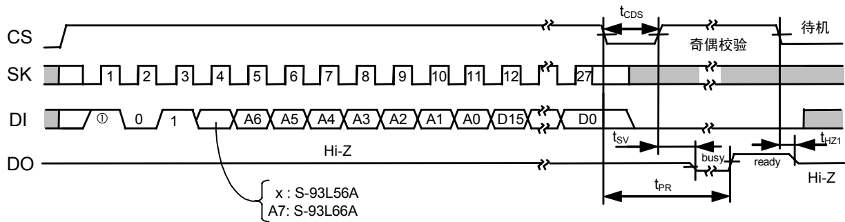
图10 数据写入定时(S-93L56A、S-93L66A)
