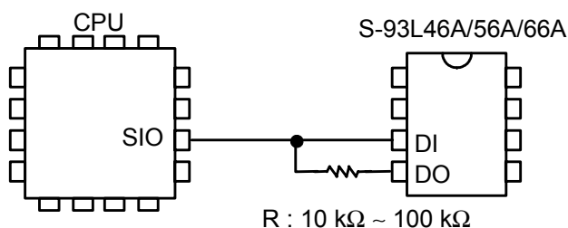
图21 3线式接口的连接法
