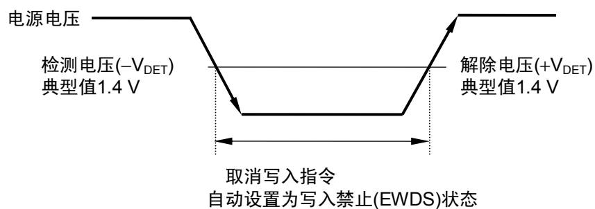
图19 低电压电源时的工作
