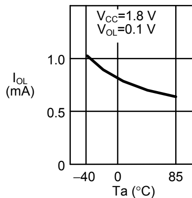
1.28 低电位输出电流 I_{OL} —周围温度 T_a
