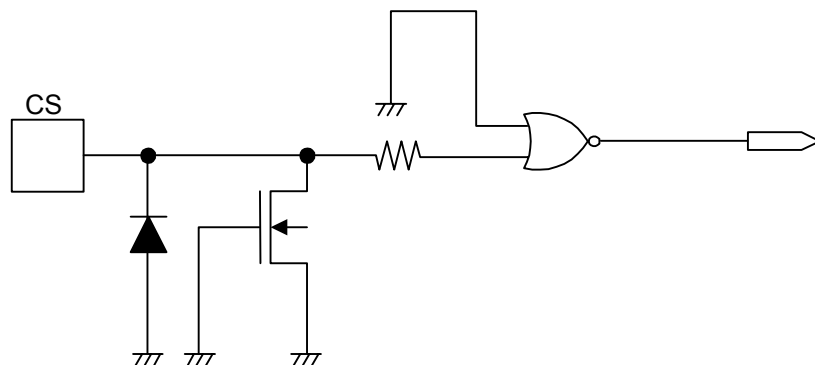
图22 CS端子
