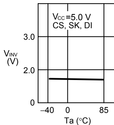
1.30 输入翻转电压 V_{INV} —周围温度 T_a
