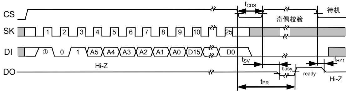
图9 数据写入定时(S-93L46A)
