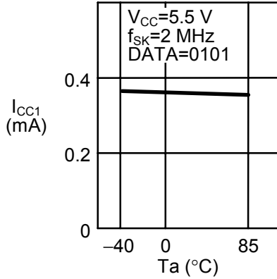
1.1 读出时消耗电流 I_{CC1} —周围温度 T_a
