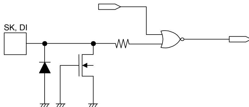
图23 SK, DI端子
