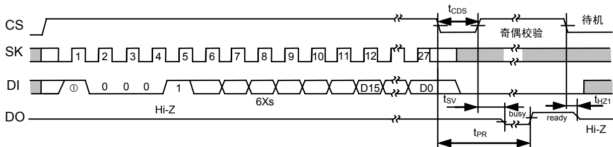
图14 全部写入定时(S-93L56A、S-93L66A)
