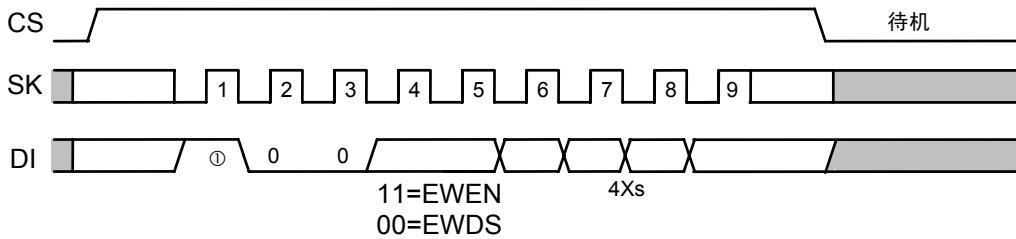
图17 写入允许 / 禁止定时(S-93L46A)
