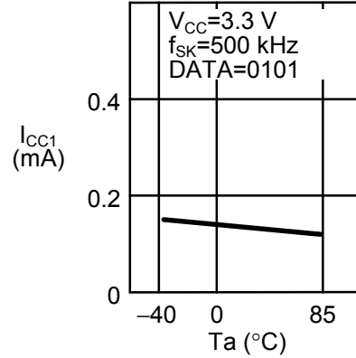
1.2 读出时消耗电流 I_{CC1} —周围温度 T_a
