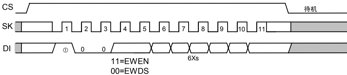
图18 写入允许 / 禁止定时(S-93L56A、S-93L66A)
