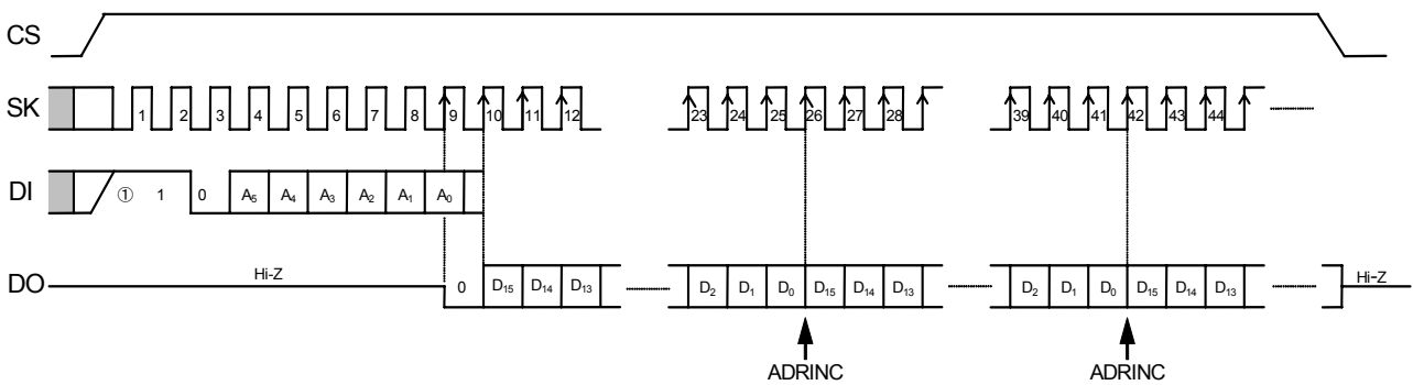
图7 读出定时(S-93L46A)
