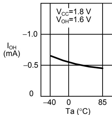
1.26 高电位输出电流 I_{OH} —周围温度 T_a
