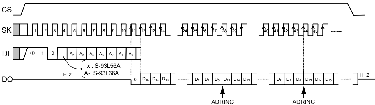
图8 读出定时(S-93L56A、S-93L66A)
