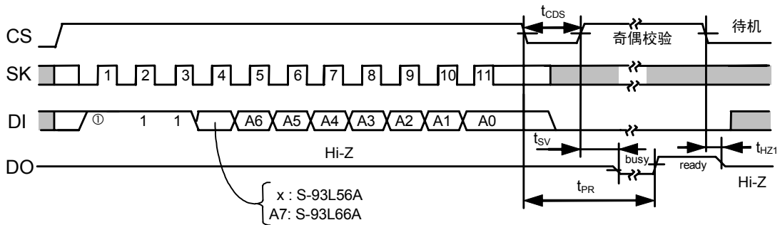
图12 数据删除定时(S-93L56A、S-93L66A)
