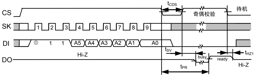
图11 数据删除定时(S-93L46A)
