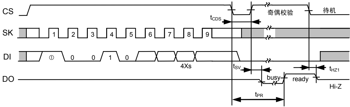
图15 全部删除定时(S-93L46A)
