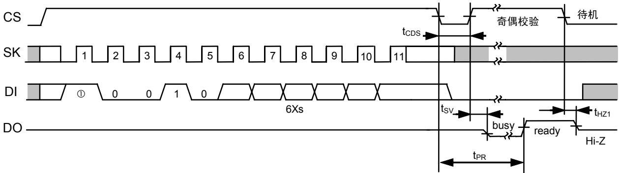
图16 全部删除定时(S-93L56A、S-93L66A)
