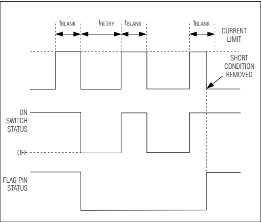
图2. MAX4796/MAX4798 自动重试故障屏蔽时序图
