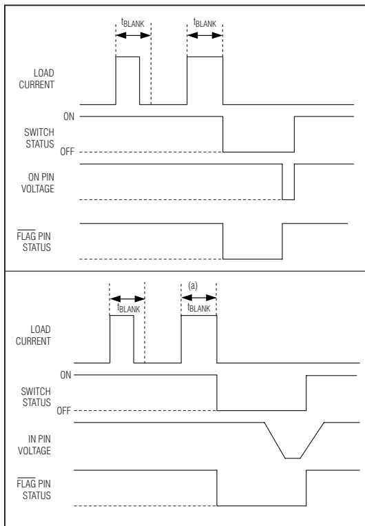
图 3. MAX4795/MAX4797 闭锁故障屏蔽
