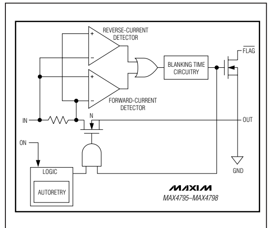
图1. 原理框图
