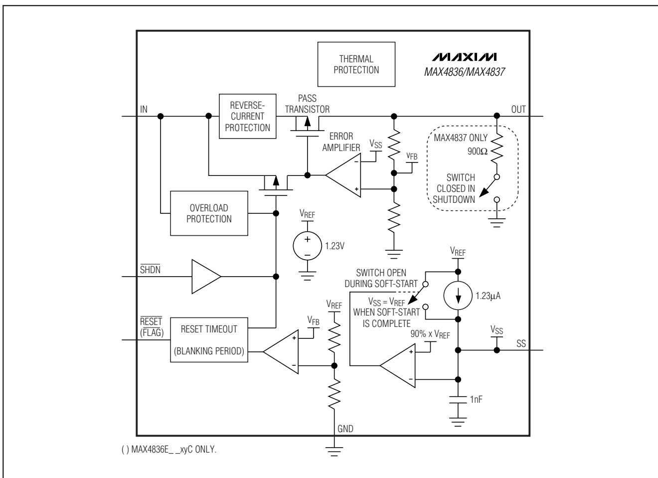
图 1. 功能框图
