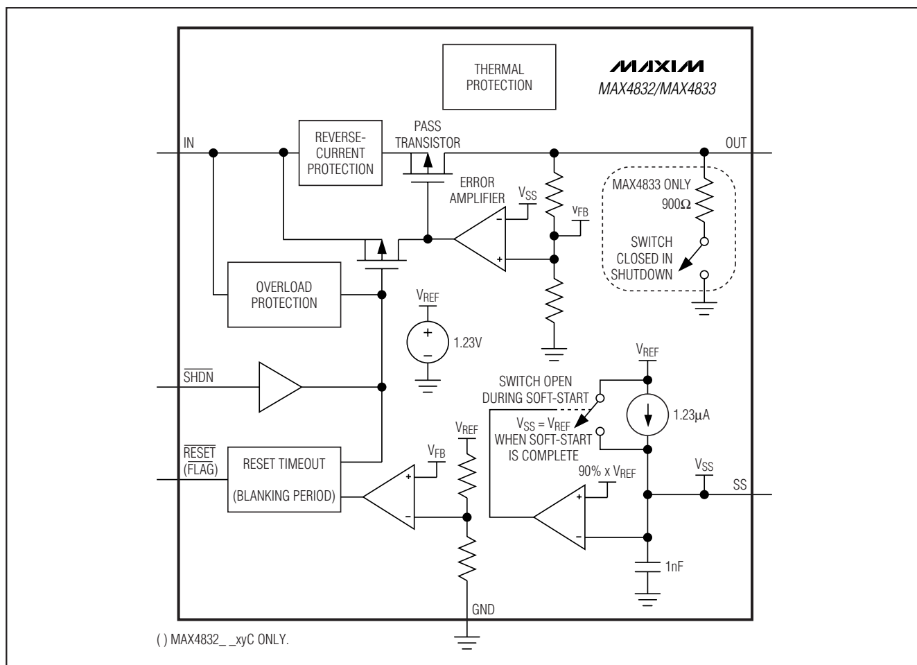
图 1. 功能框图
