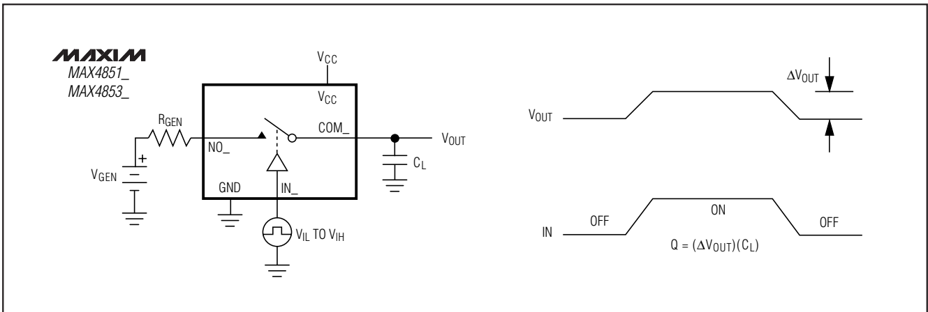
图 3. 电荷注入
