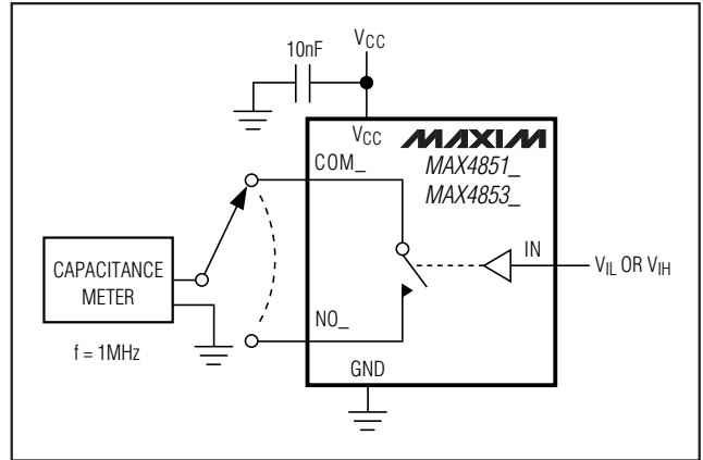
图 5. 通道关/开电容
