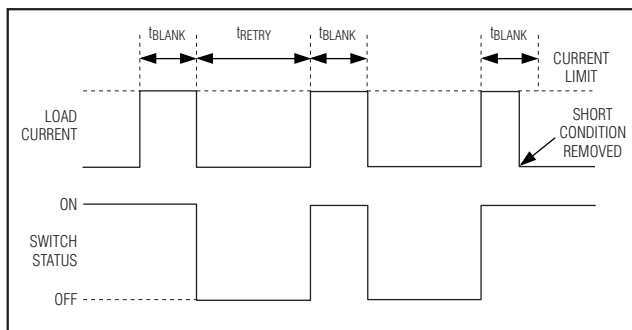
图2. MAX4827/MAX4829/MAX4831 自动重试故障屏蔽时序
