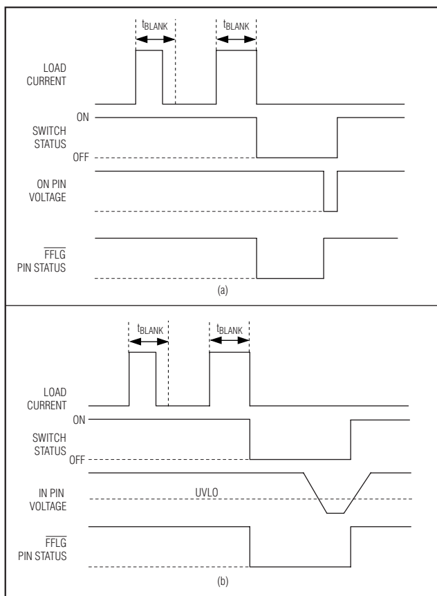
图3. MAX4826/MAX4828/MAX4830 闭锁故障屏蔽时序
