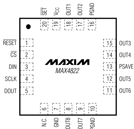
THIN QFN
