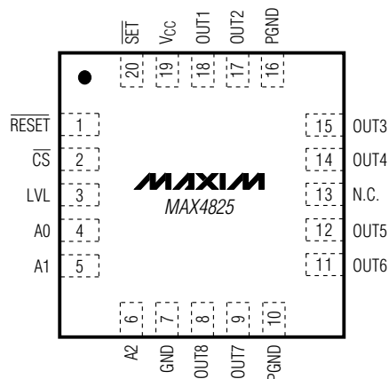
THIN QFN
